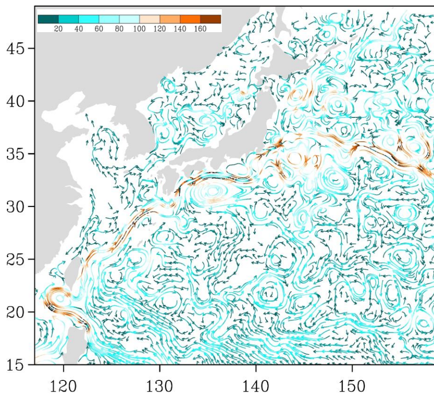
Рис. 3-6 Поверхностные течения западной части Тихого океана, 25 января 2017 г.
