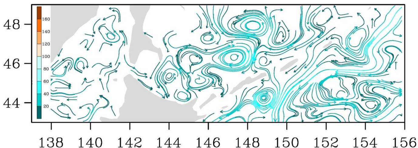
Рис. 3-9 Поверхностные течения, пролив Лаперуза, 25 января 2017 г.
