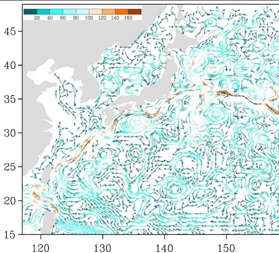
Рис. 3-5 Поверхностные течения западной части Тихого океана, 15 января 2017 г.
