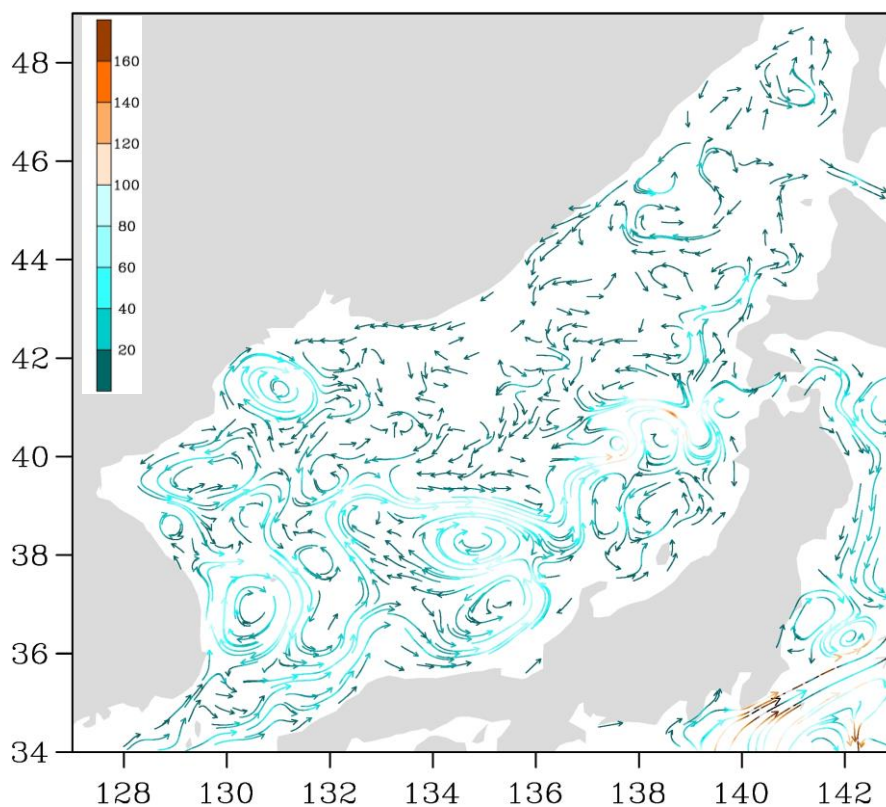
Рис. 3-3 Поверхностные течения Японского моря, 25 января 2017 г.
