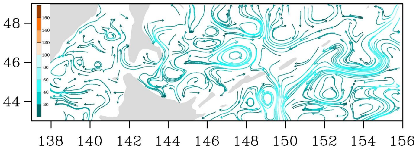
Рис. 3-8 Поверхностные течения, пролив Лаперуза, 15 января 2017 г.
