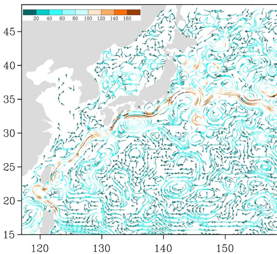
Рис. 3-4 Поверхностные течения западной части Тихого океана, 5 января 2017 г.
