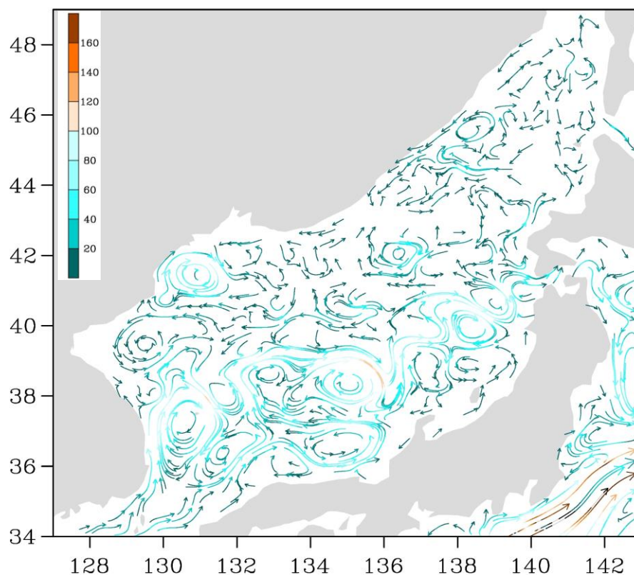
Рис. 3-1 Поверхностные течения Японского моря, 05 января 2017 г.
