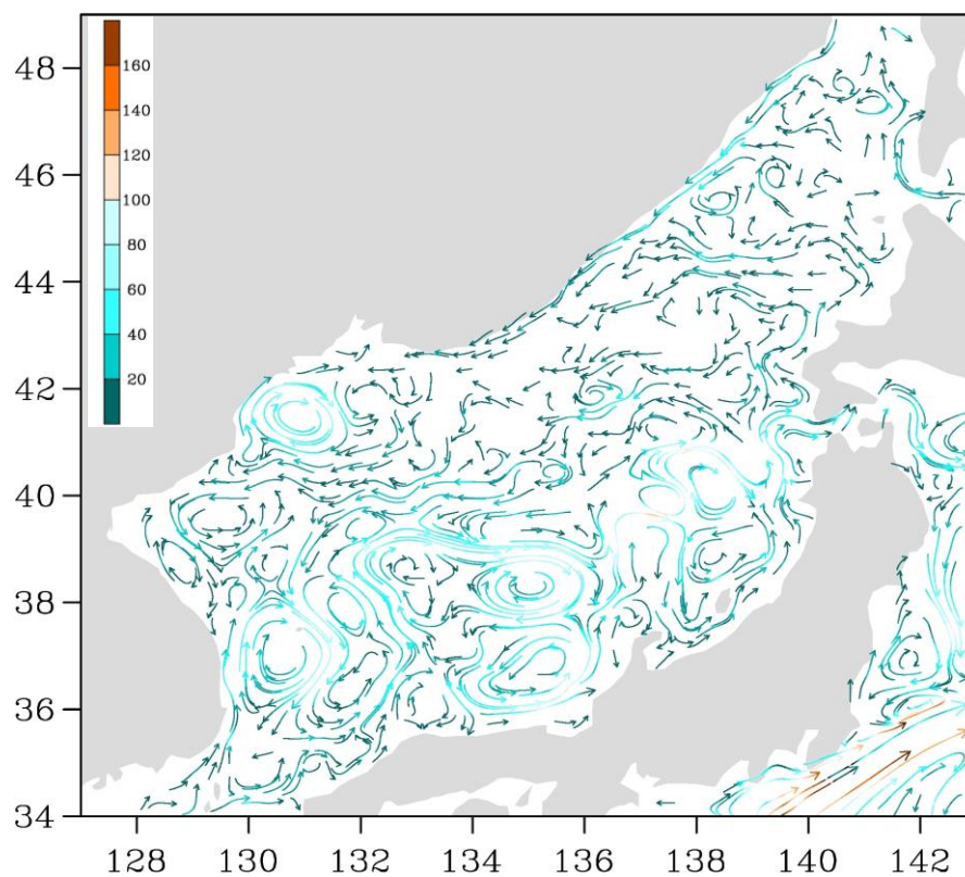
Рис. 3-2 Поверхностные течения Японского моря, 15 января 2017 г.
