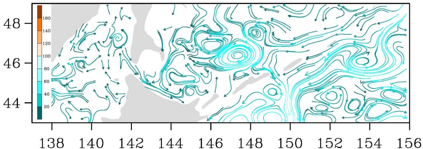
Рис. 3-7 Поверхностные течения, пролив Лаперуза, 5 января 2017 г.
