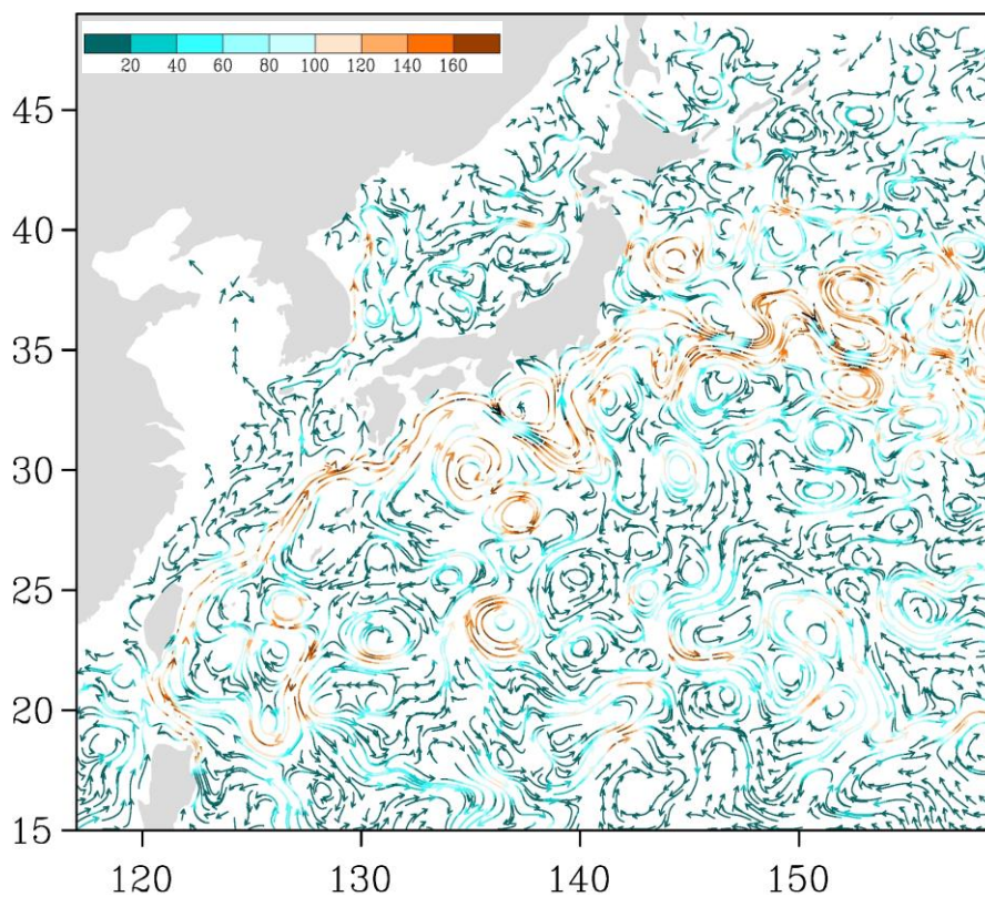
Рис. 3-6 Поверхностные течения западной части Тихого океана, 25 октября 2017 г.
