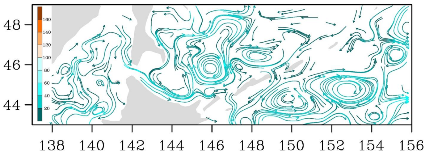
Рис. 3-9 Поверхностные течения, пролив Лаперуза, 25 октября 2017 г.
