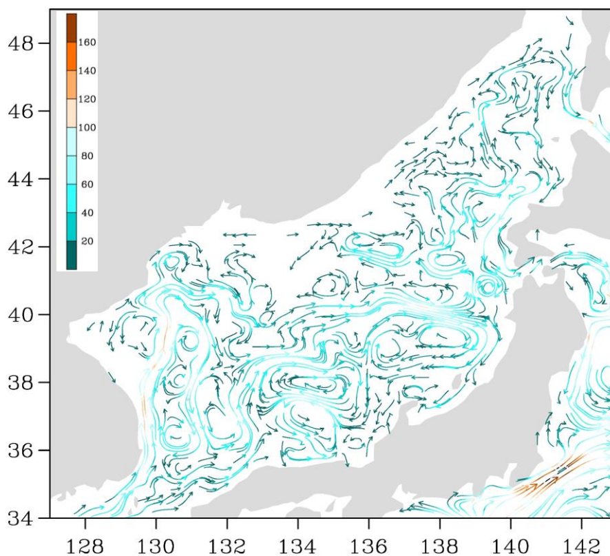
Рис. 3-3 Поверхностные течения Японского моря, 25 октября 2017 г.
