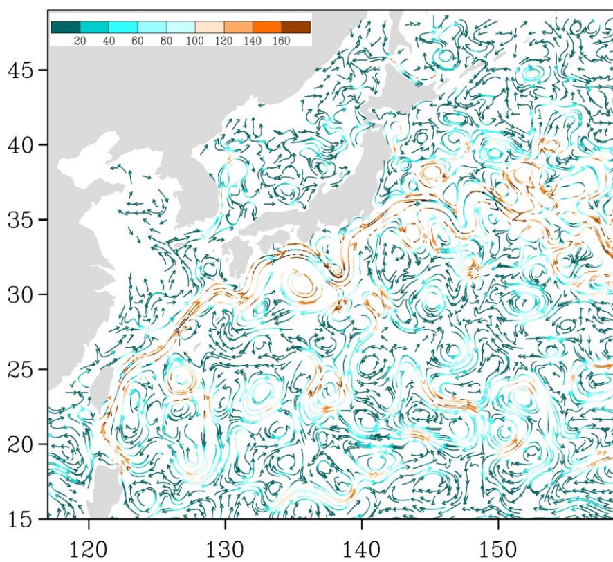
Рис. 3-4 Поверхностные течения западной части Тихого океана, 5 октября 2017 г.
