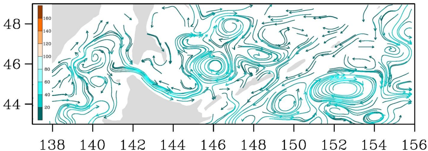
Рис. 3-8 Поверхностные течения, пролив Лаперуза, 15 октября 2017 г.
