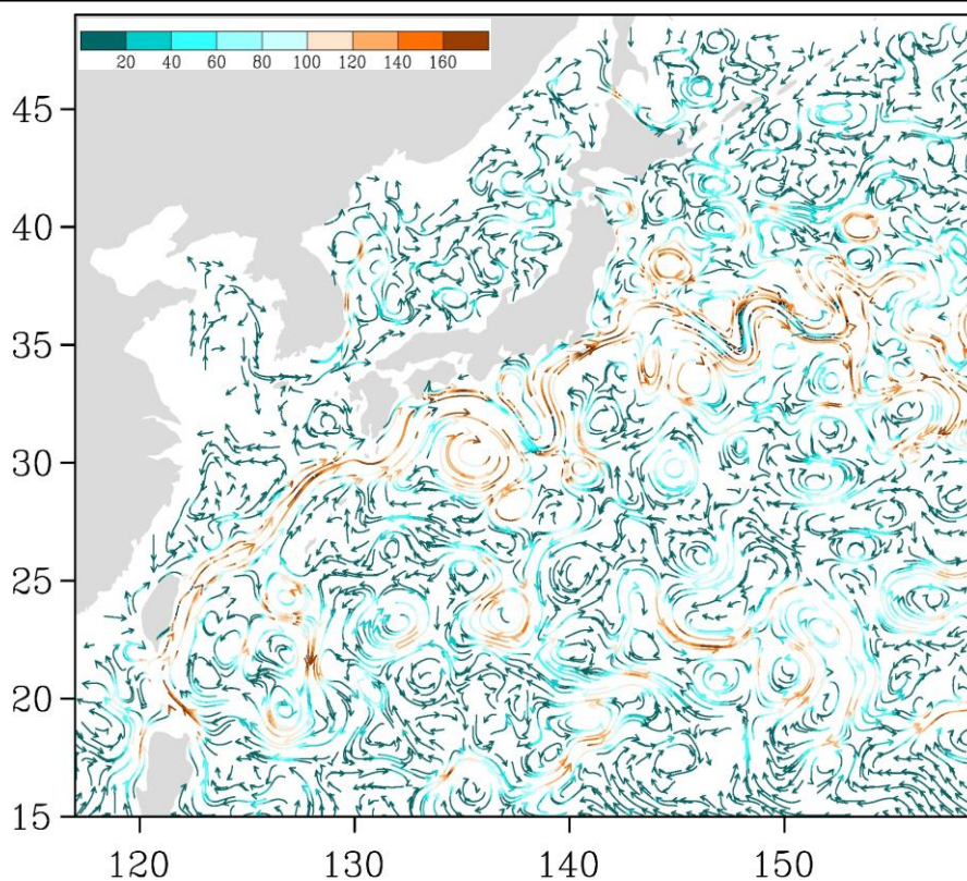
Рис. 3-5 Поверхностные течения западной части Тихого океана, 15 октября 2017 г.
