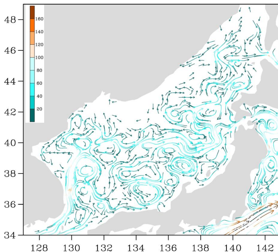
Рис. 3-1 Поверхностные течения Японского моря, 05 октября 2017 г.
