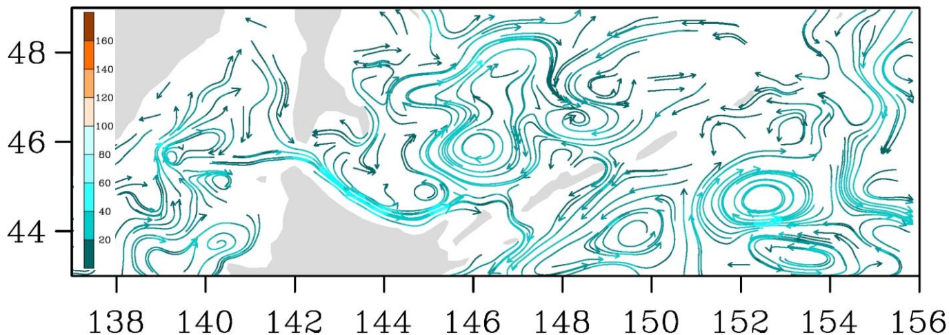
Рис. 3-7 Поверхностные течения, пролив Лаперуза, 5 октября 2017 г.
