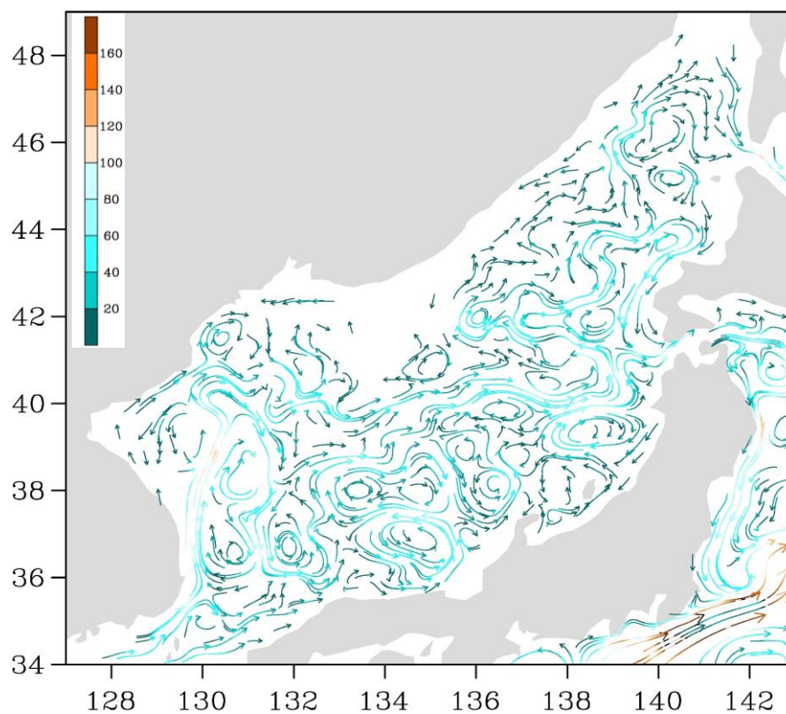
Рис. 3-2 Поверхностные течения Японского моря, 15 октября 2017 г.
