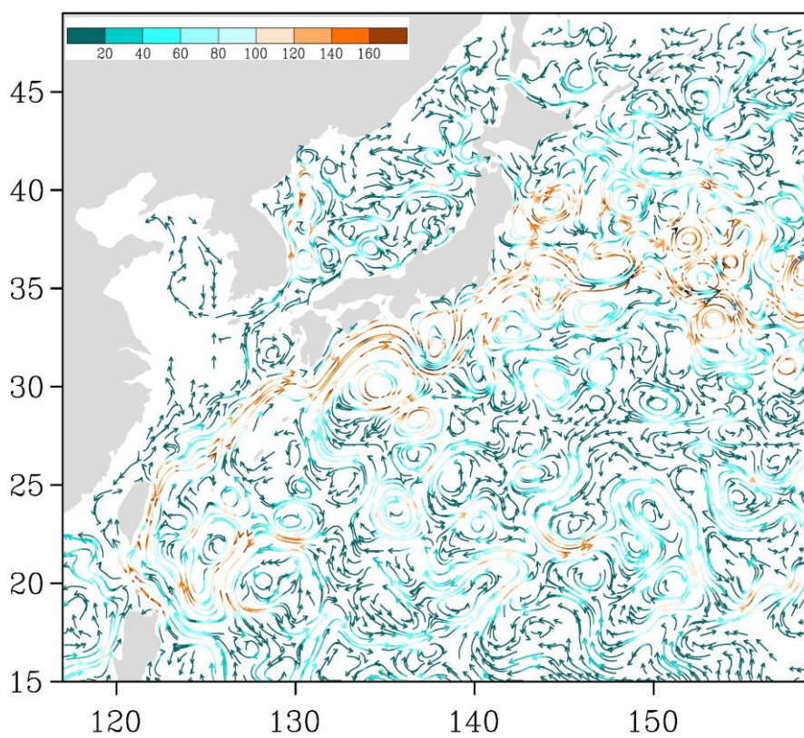
Рис. 3-4 Поверхностные течения западной части Тихого океана, 5 ноября 2017 г.
