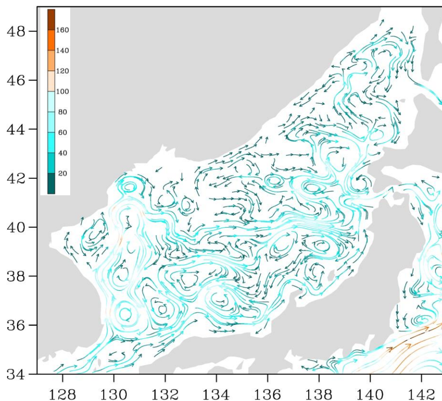
Рис. 3-1 Поверхностные течения Японского моря, 05 ноября 2017 г.
