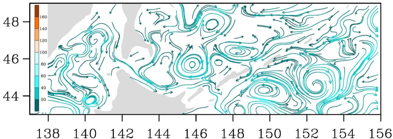
Рис. 3-7 Поверхностные течения, пролив Лаперуза, 5 ноября 2017 г.
