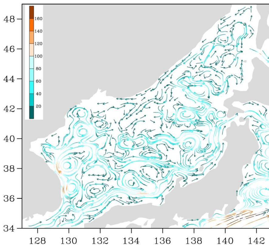
Рис. 3-3 Поверхностные течения Японского моря, 25 ноября 2017 г.
