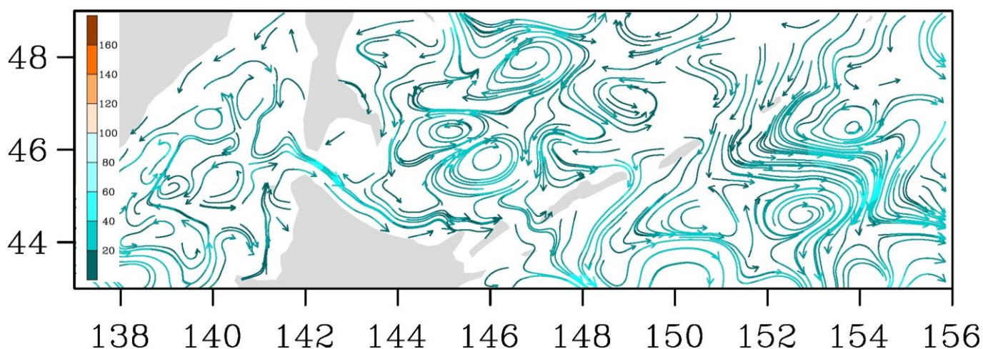
Рис. 3-9 Поверхностные течения, пролив Лаперуза, 25 ноября 2017 г.
