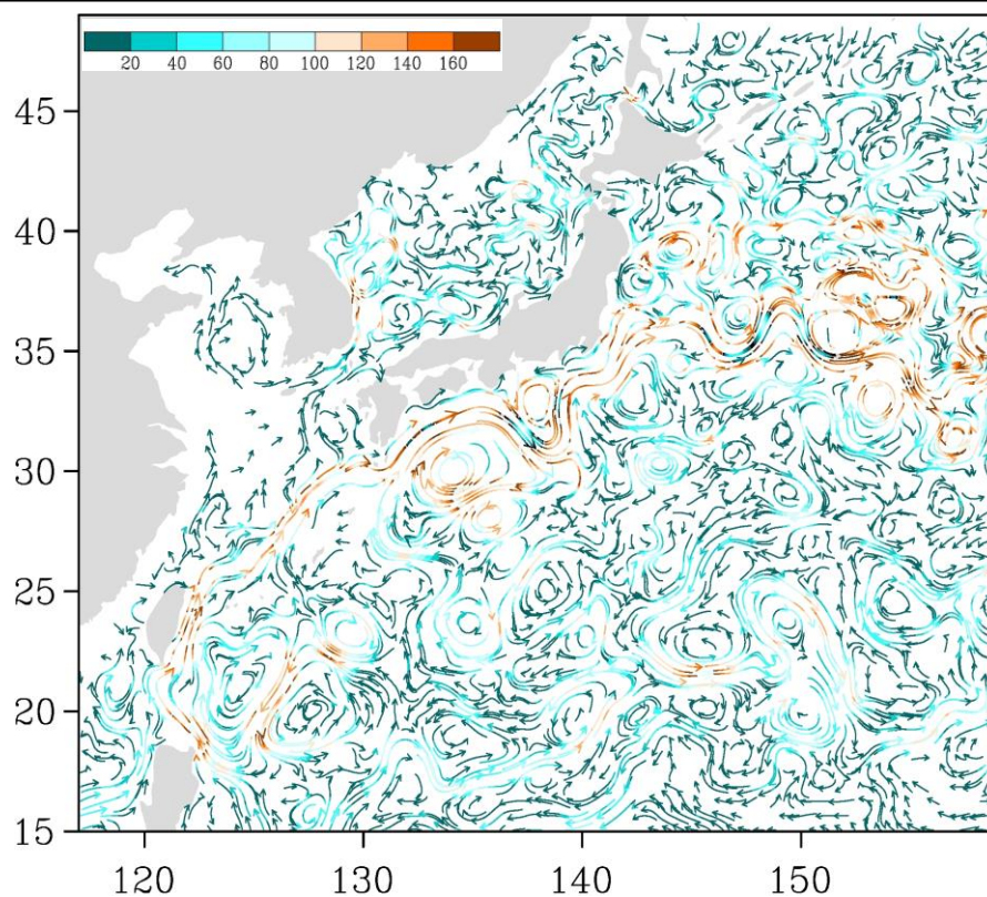
Рис. 3-5 Поверхностные течения западной части Тихого океана, 15 ноября 2017 г.
