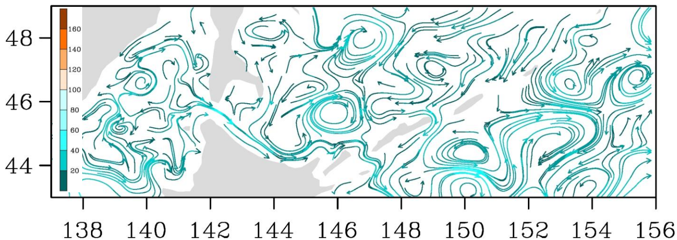
Рис. 3-8 Поверхностные течения, пролив Лаперуза, 15 ноября 2017 г.
