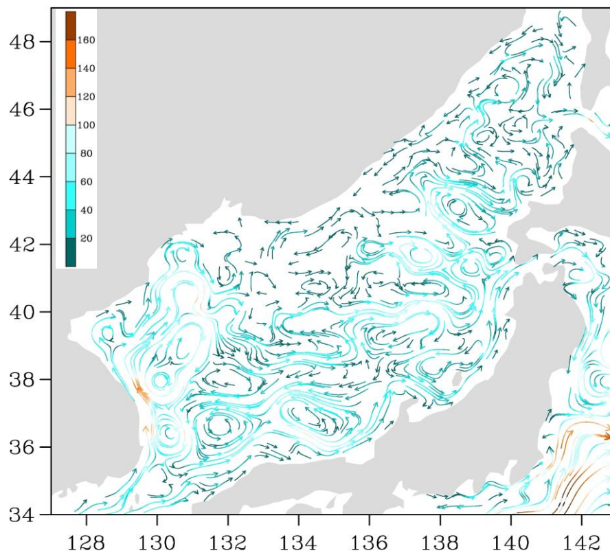
Рис. 3-2 Поверхностные течения Японского моря, 15 ноября 2017 г.
