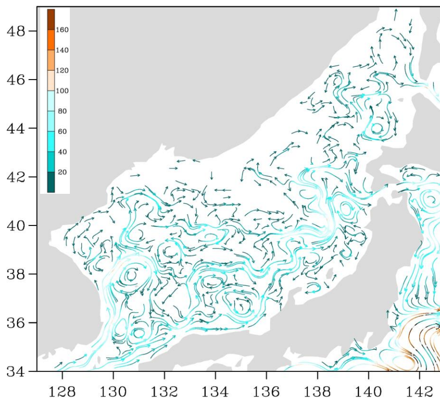
Рис. 3-1 Поверхностные течения Японского моря, 05 сентября 2017 г.
