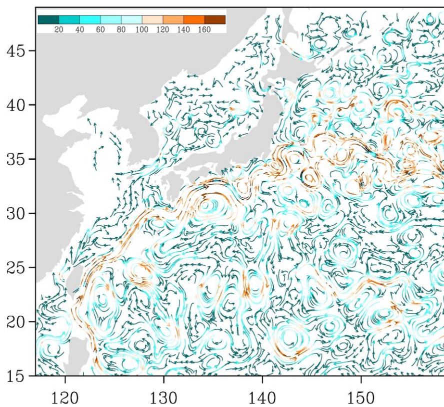
Рис. 3-4 Поверхностные течения западной части Тихого океана, 5 сентября 2017 г.
