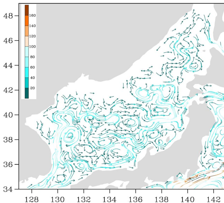
Рис. 3-3 Поверхностные течения Японского моря, 25 сентября 2017 г.
