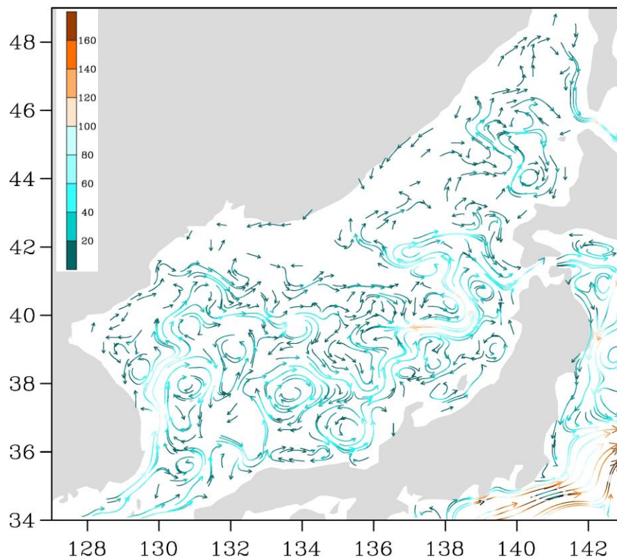
Рис. 3-2 Поверхностные течения Японского моря, 15 сентября 2017 г.
