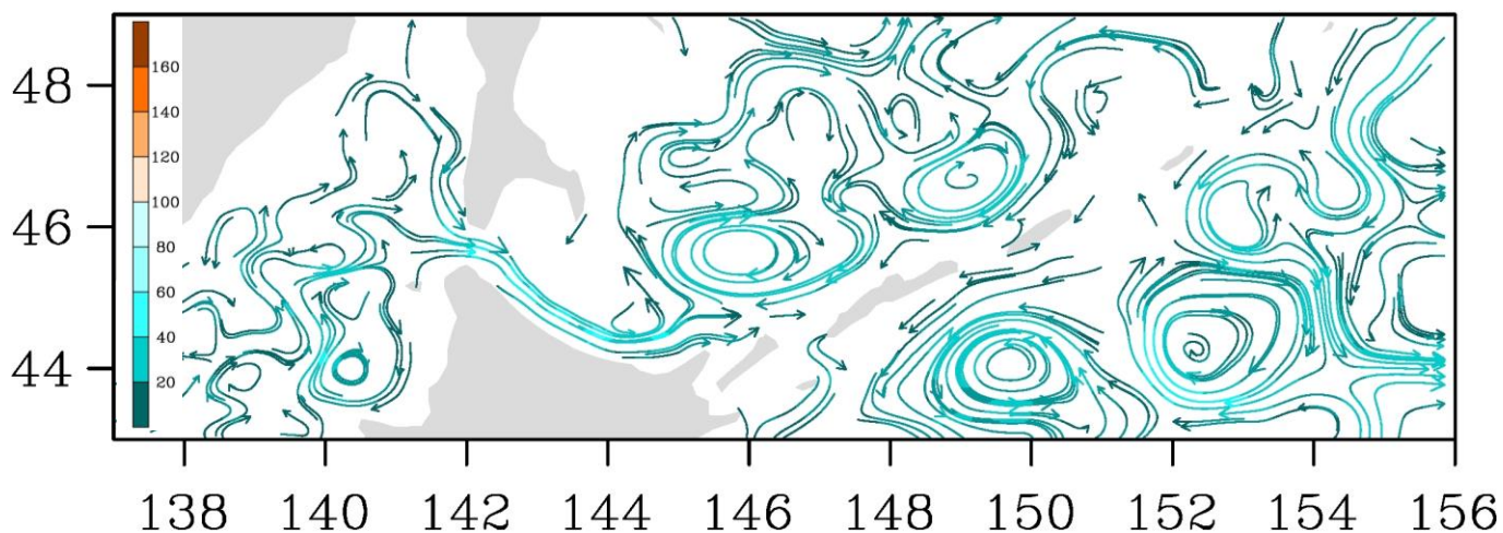
Рис. 3-7 Поверхностные течения, пролив Лаперуза, 5 сентября 2017 г.
