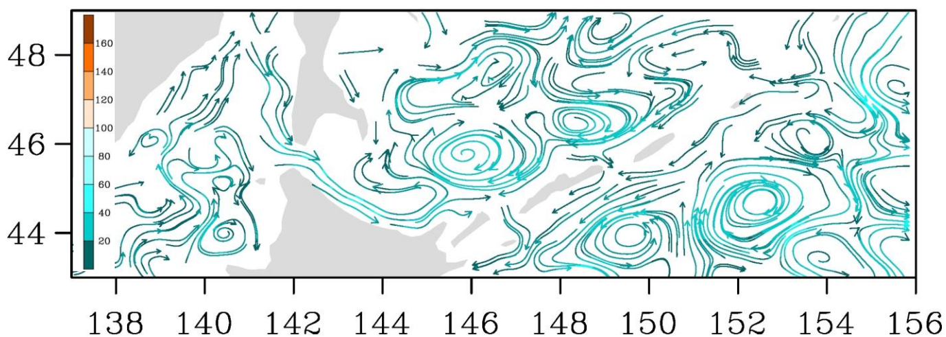
Рис. 3-9 Поверхностные течения, пролив Лаперуза, 25 сентября 2017 г.
