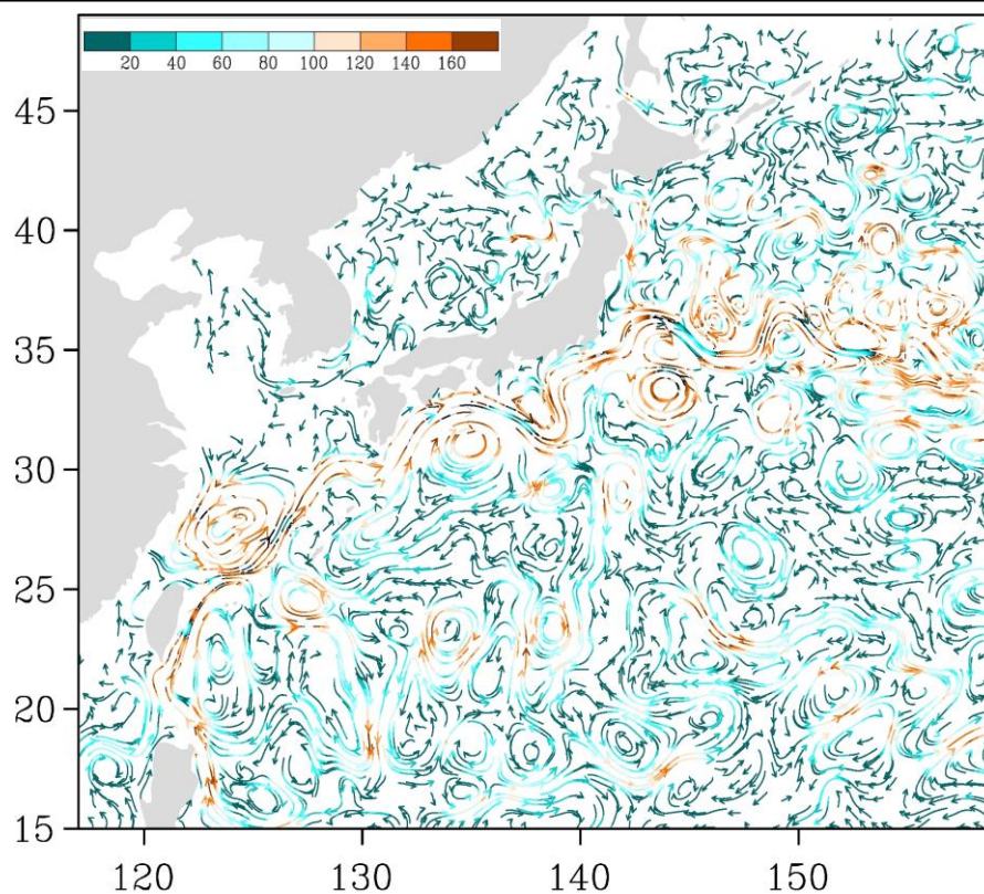
Рис. 3-5 Поверхностные течения западной части Тихого океана, 15 сентября 2017 г.
