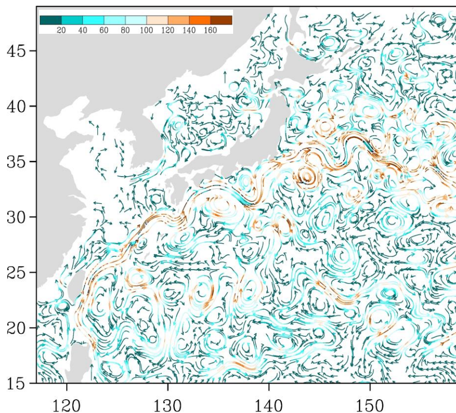
Рис. 3-6 Поверхностные течения западной части Тихого океана, 25 сентября 2017 г.
