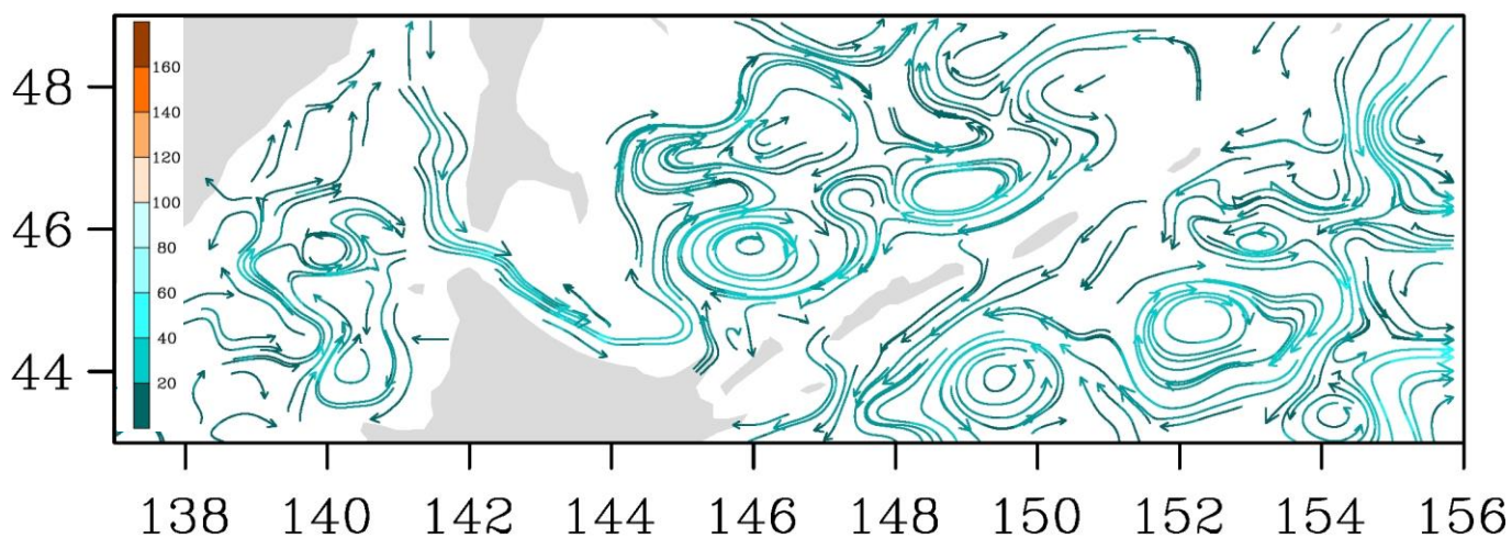
Рис. 3-8 Поверхностные течения, пролив Лаперуза, 15 сентября 2017 г.
