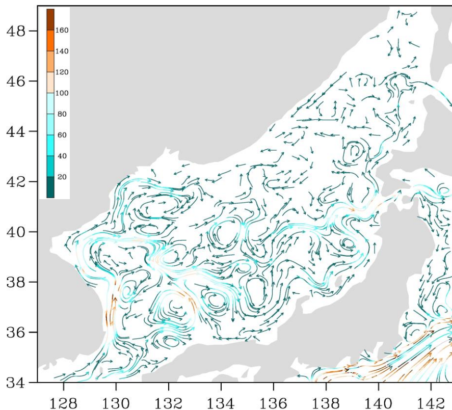
Рис. 3-2 Поверхностные течения Японского моря, 15 декабря 2019 г.
