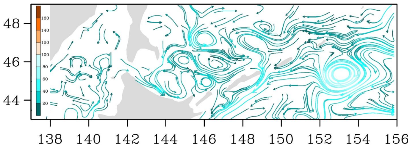
Рис. 3-8 Поверхностные течения, пролив Лаперуза, 15 декабря 2019 г.
