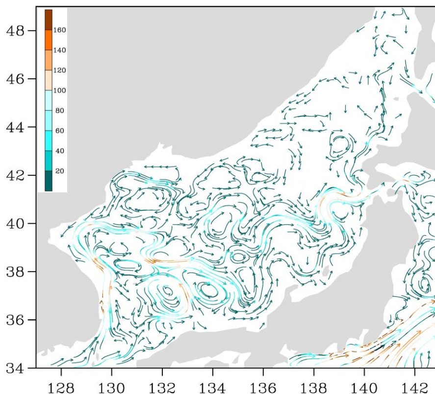
Рис. 3-3 Поверхностные течения Японского моря, 25 декабря 2019 г.
