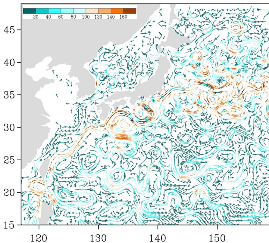
Рис. 3-5 Поверхностные течения западной части Тихого океана, 15 декабря 2019 г.
