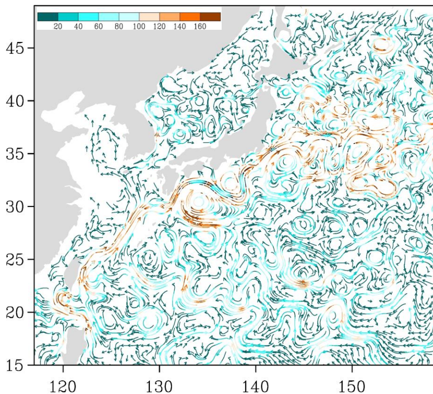
Рис. 3-4 Поверхностные течения западной части Тихого океана, 5 декабря 2019 г.
