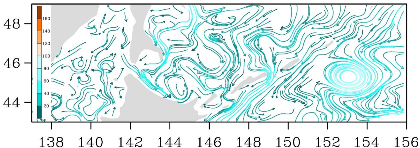
Рис. 3-7 Поверхностные течения, пролив Лаперуза, 5 декабря 2019 г.
