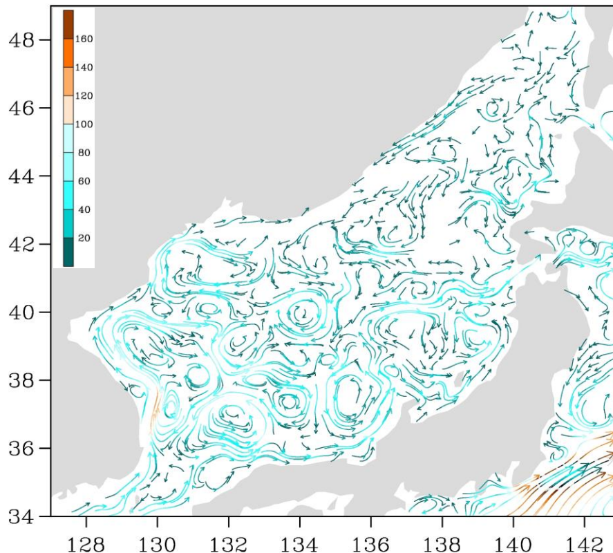
Рис. 3-1 Поверхностные течения Японского моря, 05 декабря 2019 г.
