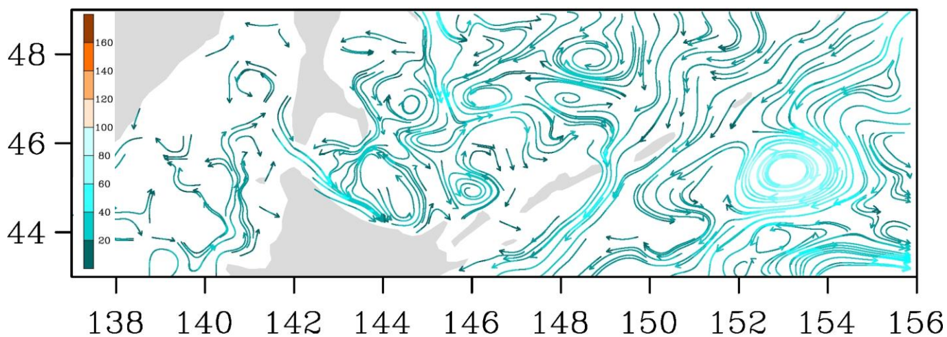
Рис. 3-9 Поверхностные течения, пролив Лаперуза, 25 декабря 2019 г.
