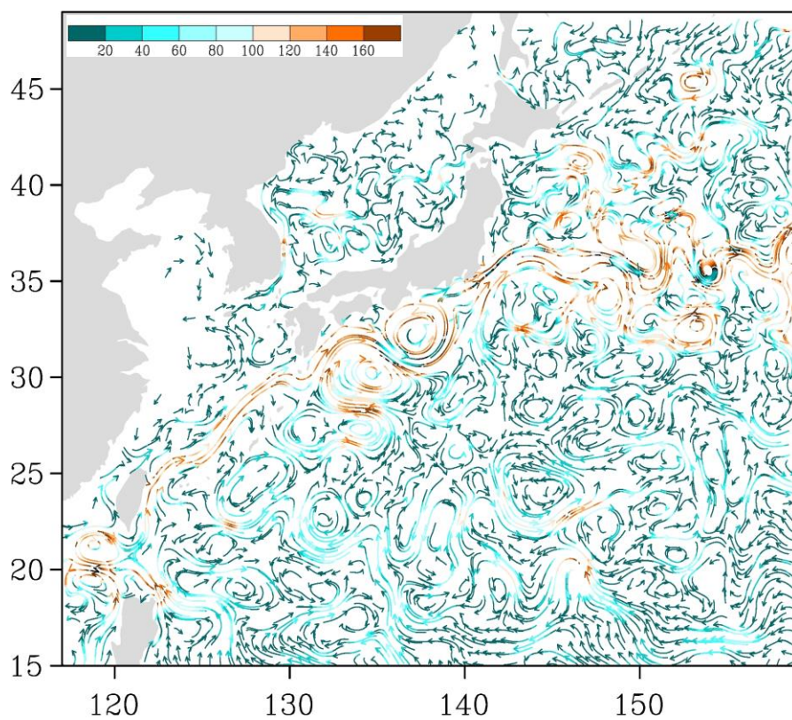
Рис. 3-6 Поверхностные течения западной части Тихого океана, 25 декабря 2019 г.
