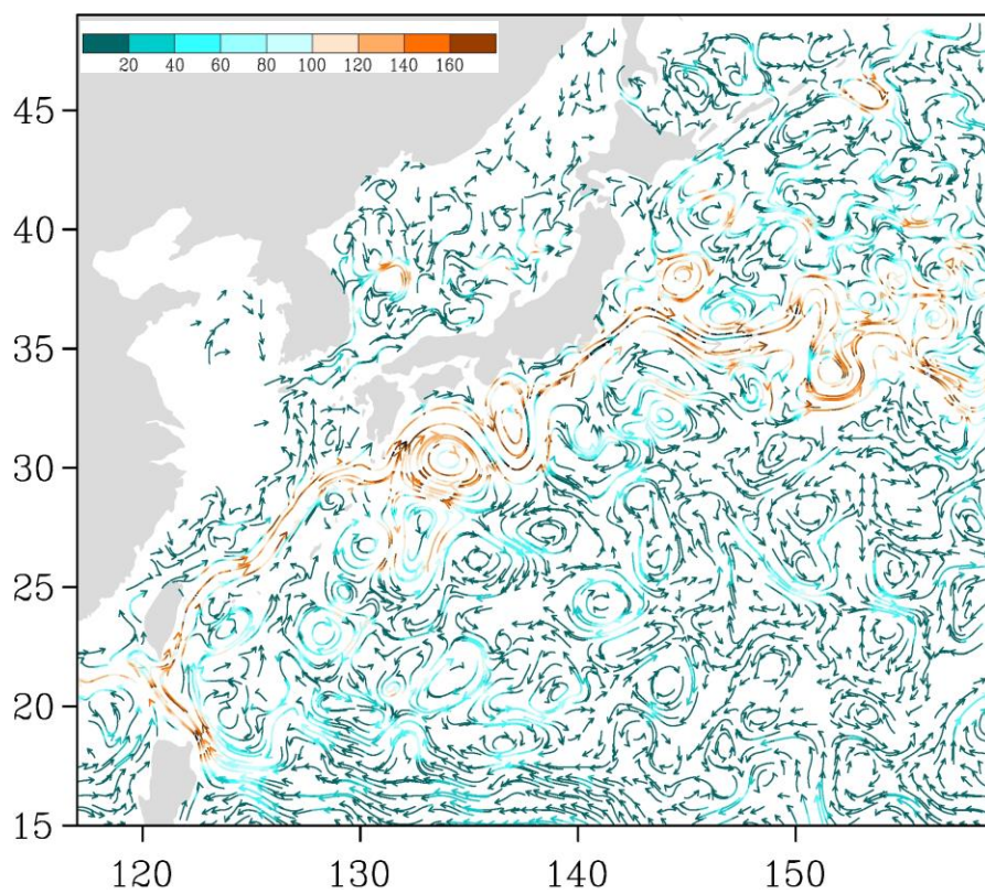
Рис. 3-6 Поверхностные течения западной части Тихого океана, 25 февраля 2019 г.
