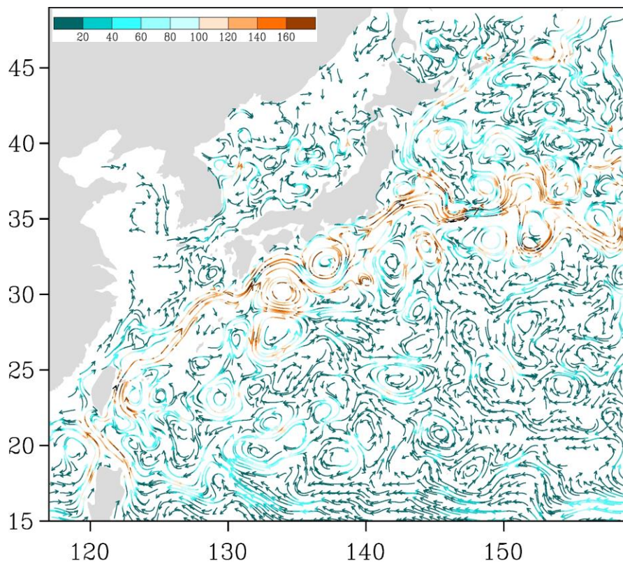
Рис. 3-4 Поверхностные течения западной части Тихого океана, 5 февраля 2019 г.
