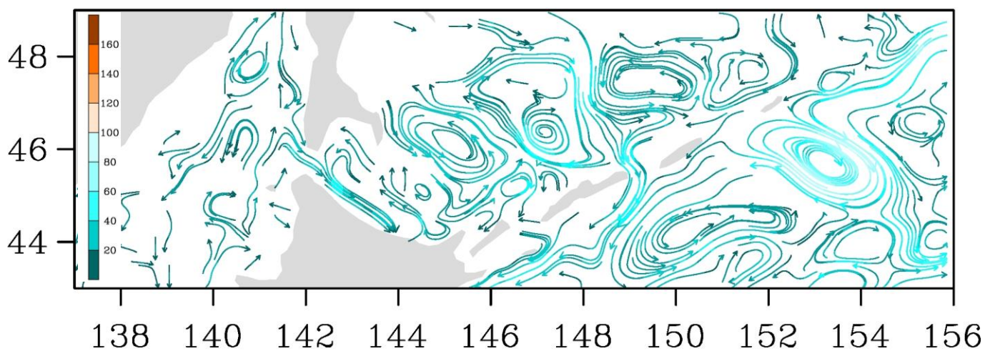
Рис. 3-9 Поверхностные течения, пролив Лаперуза, 25 февраля 2019 г.
