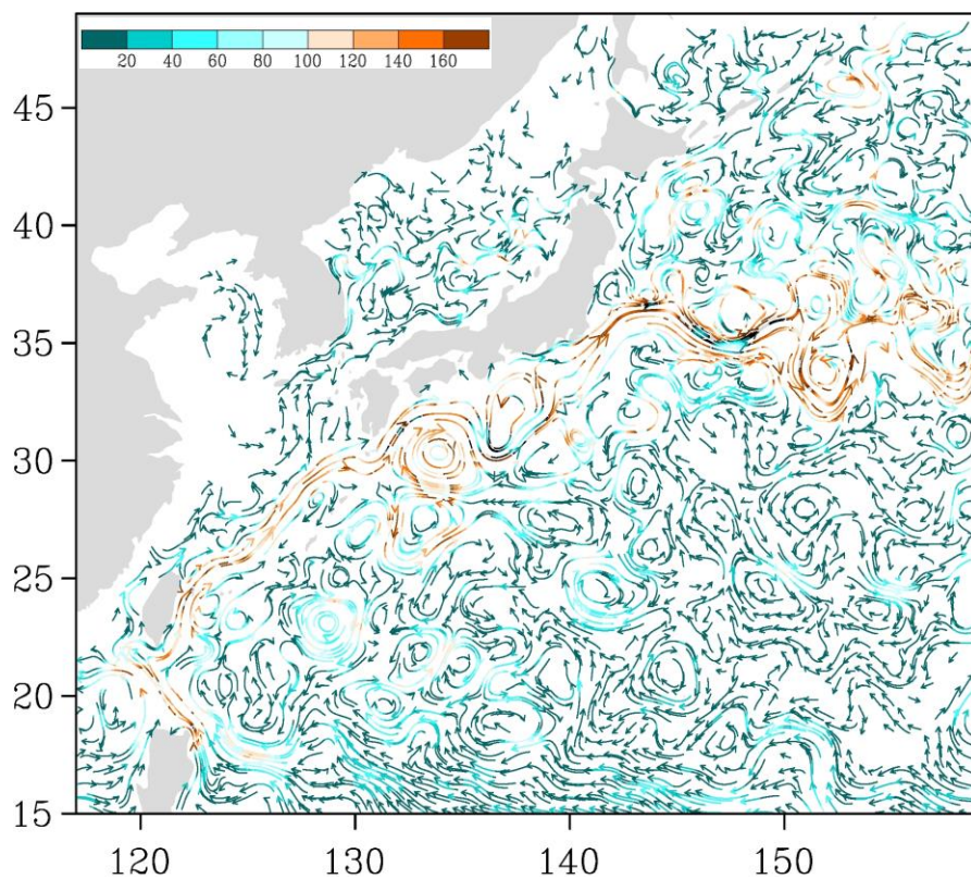
Рис. 3-5 Поверхностные течения западной части Тихого океана, 15 февраля 2019 г.
