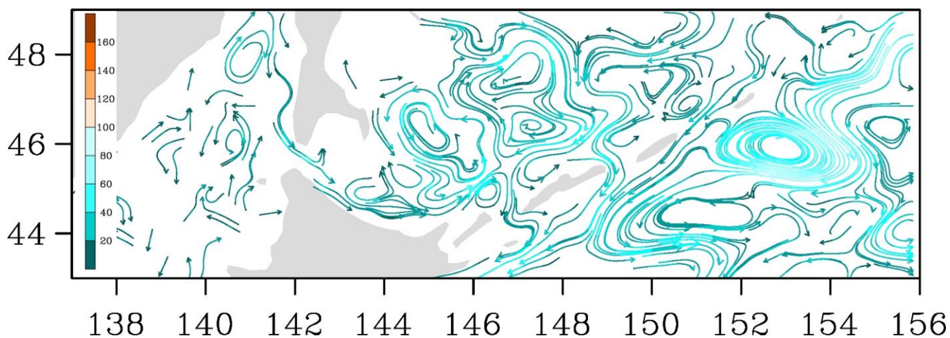
Рис. 3-8 Поверхностные течения, пролив Лаперуза, 15 февраля 2019 г.
