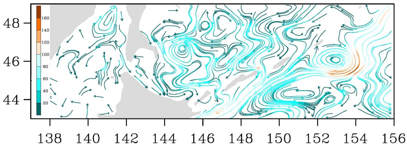
Рис. 3-7 Поверхностные течения, пролив Лаперуза, 5 февраля 2019 г.
