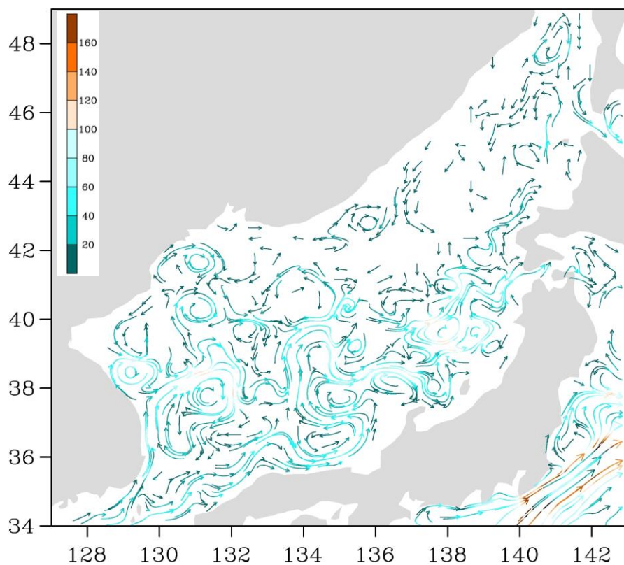
Рис. 3-3 Поверхностные течения Японского моря, 25 февраля 2019 г.
