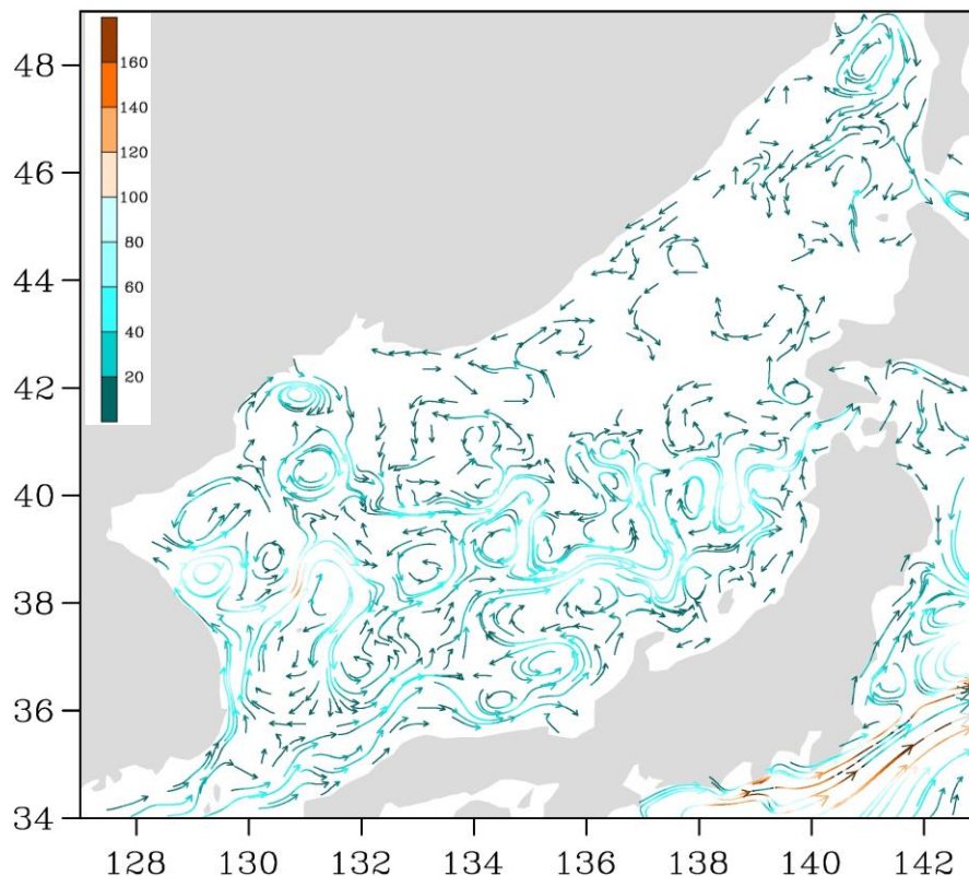
Рис. 3-1 Поверхностные течения Японского моря, 05 февраля 2019 г.
