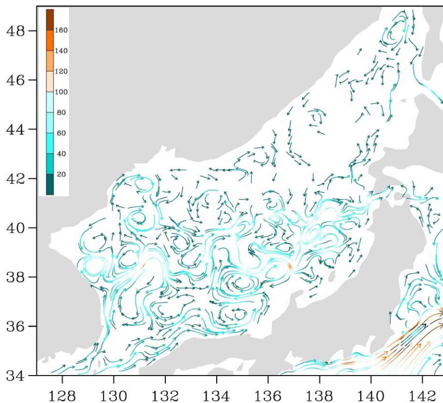
Рис. 3-2 Поверхностные течения Японского моря, 15 февраля 2019 г.
