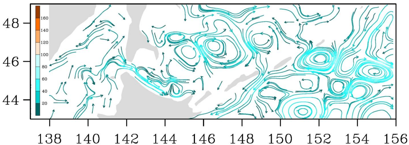
Рис. 3-7 Поверхностные течения, пролив Лаперуза, 5 июня 2019 г.
