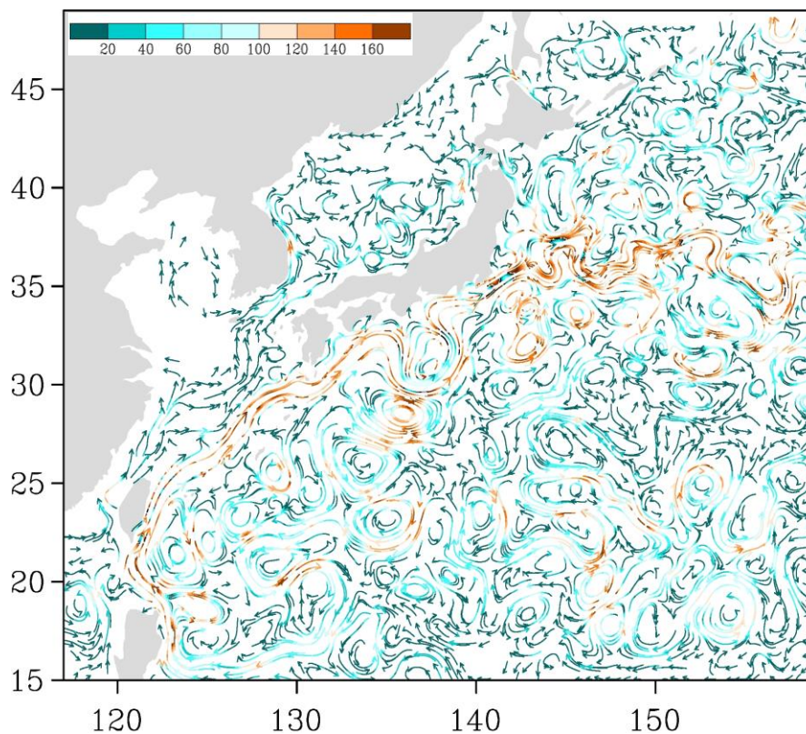
Рис. 3-4 Поверхностные течения западной части Тихого океана, 5 июня 2019 г.
