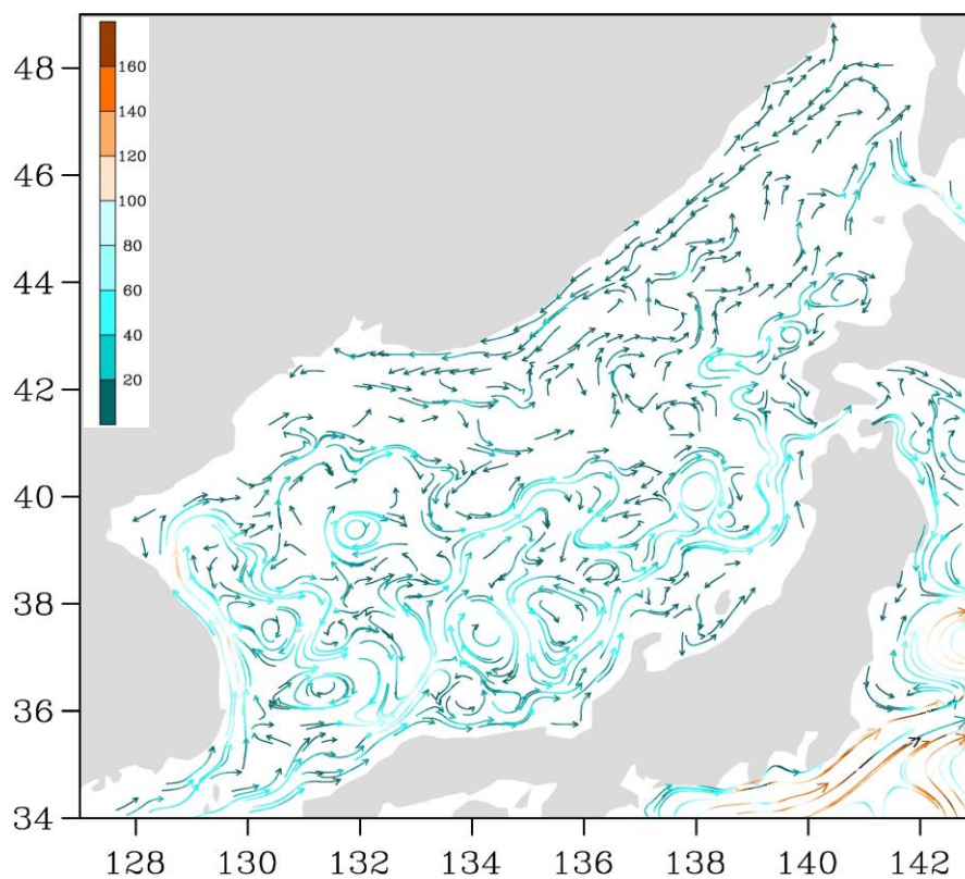
Рис. 3-3 Поверхностные течения Японского моря, 25 июня 2019 г.
