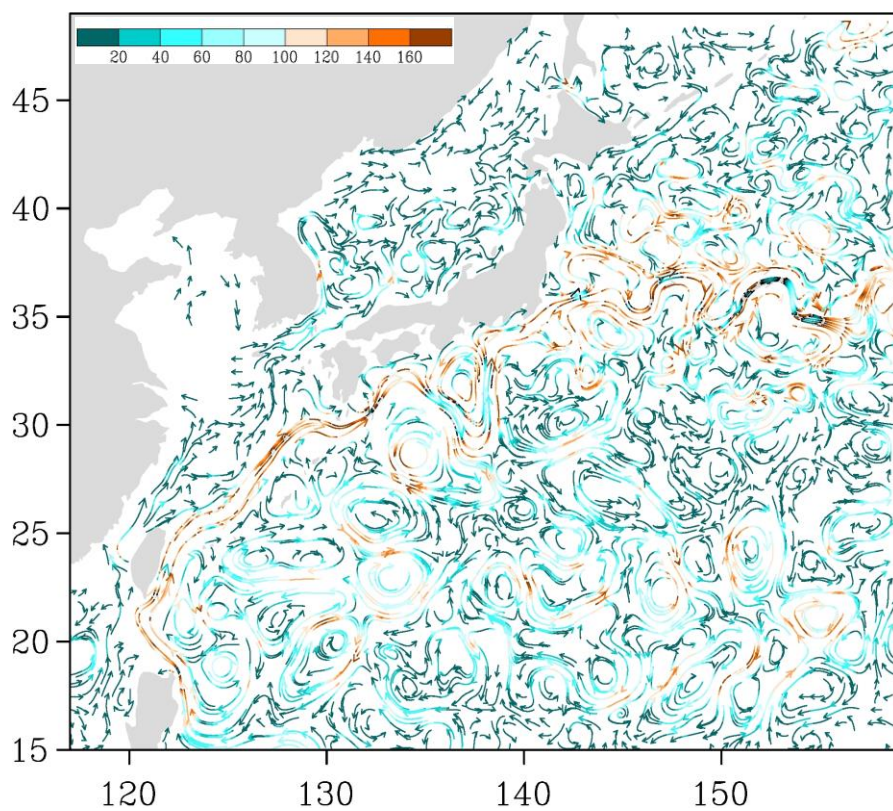
Рис. 3-6 Поверхностные течения западной части Тихого океана, 25 июня 2019 г.
