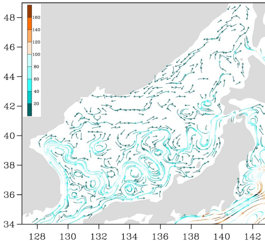
Рис. 3-1 Поверхностные течения Японского моря, 05 июня 2019 г.
