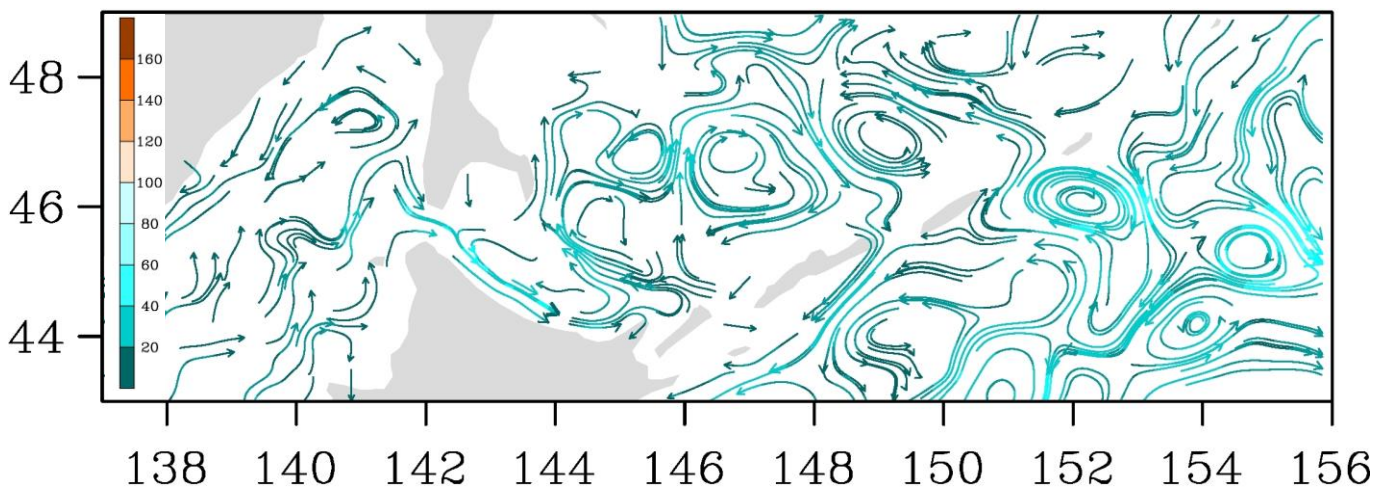
Рис. 3-8 Поверхностные течения, пролив Лаперуза, 15 июня 2019 г.
