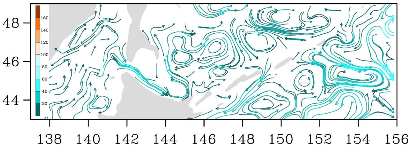
Рис. 3-9 Поверхностные течения, пролив Лаперуза, 25 июня 2019 г.
