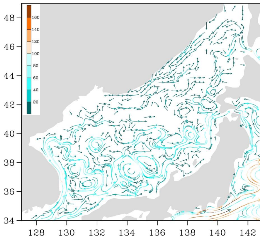
Рис. 3-2 Поверхностные течения Японского моря, 15 июня 2019 г.
