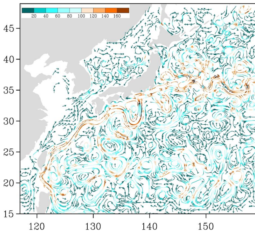
Рис. 3-5 Поверхностные течения западной части Тихого океана, 15 июня 2019 г.
