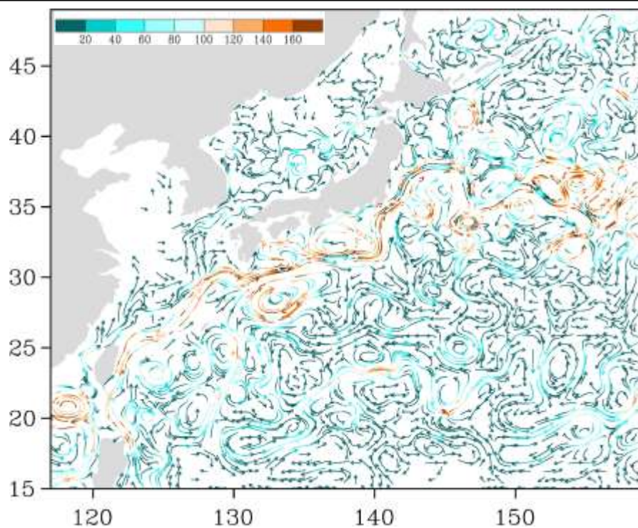
Рис. 3-5 Поверхностные течения западной части Тихого океана, 15 марта 2021 г.
