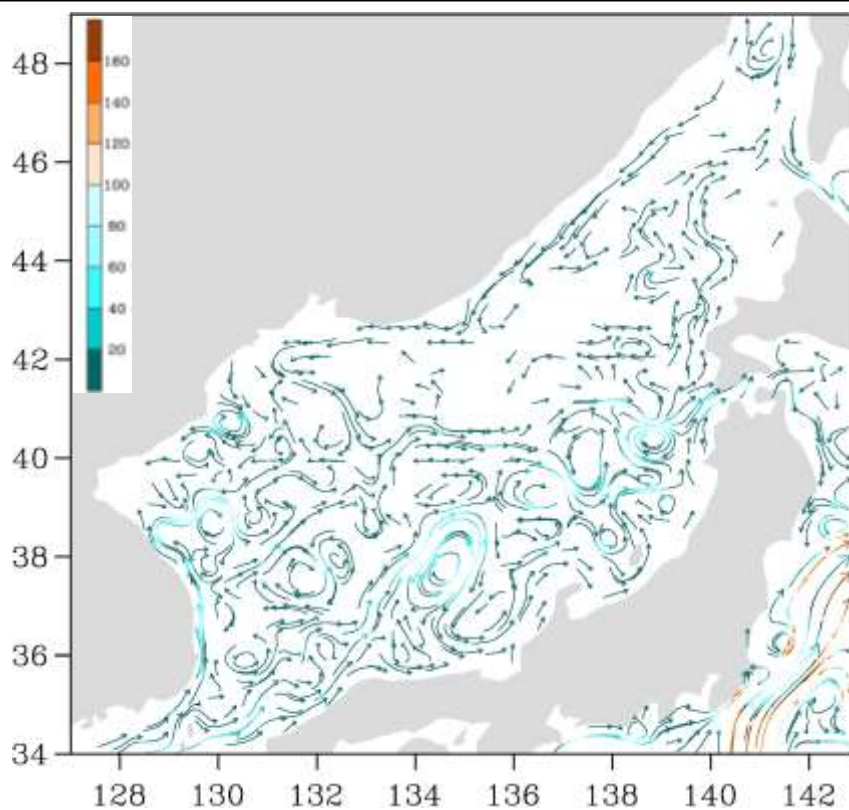
Рис. 3-3 Поверхностные течения Японского моря, 25 марта 2021 г.
