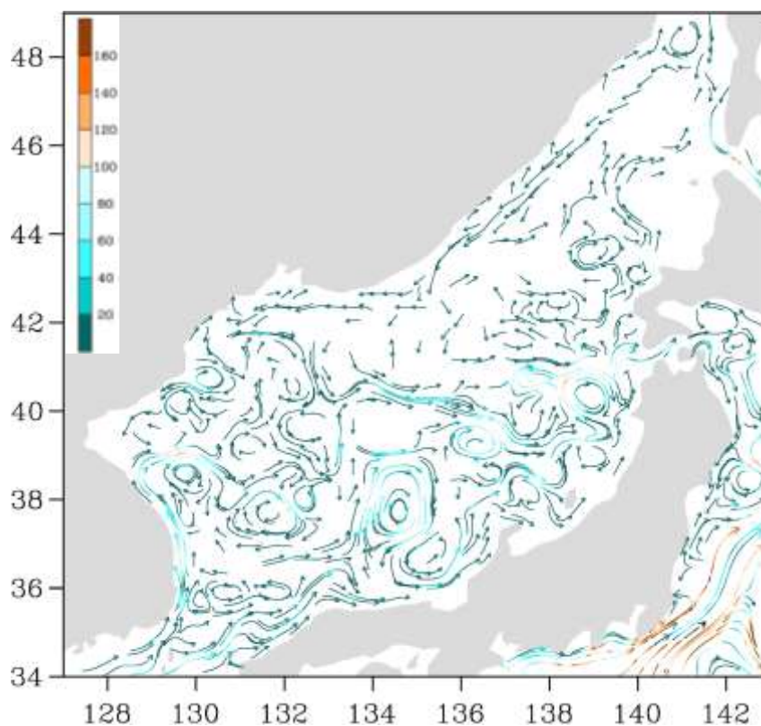
Рис. 3-2 Поверхностные течения Японского моря, 15 марта 2021 г.
