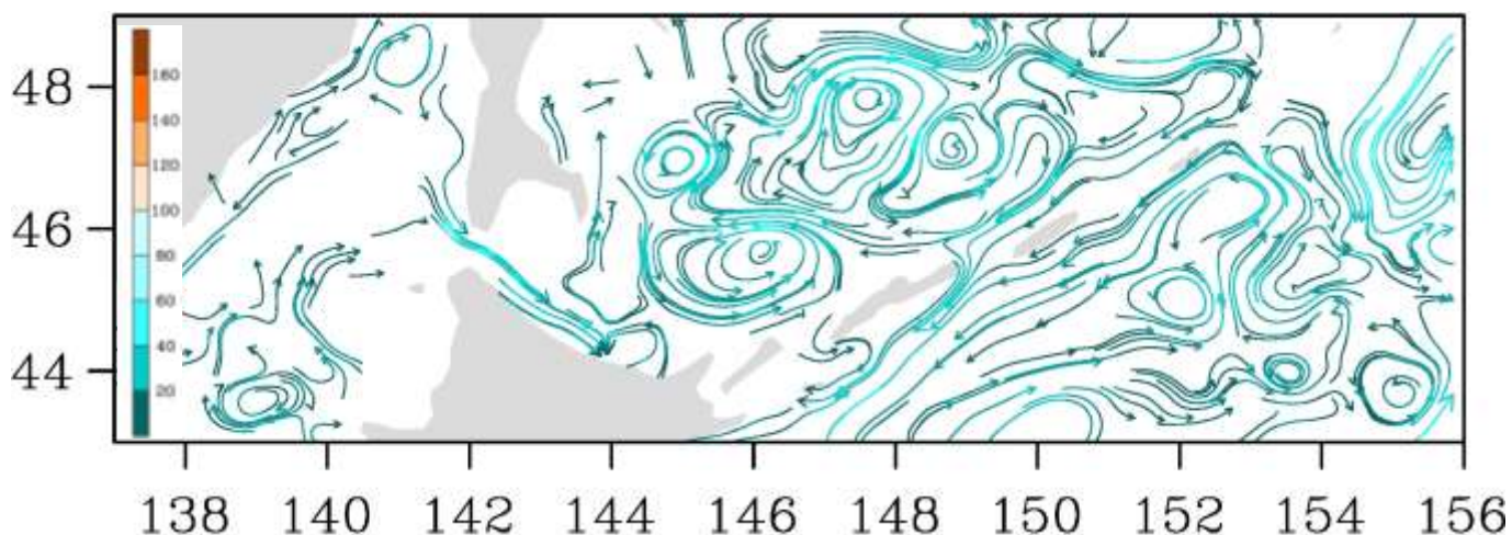
Рис. 3-8 Поверхностные течения, пролив Лаперуза, 15 марта 2021 г.
