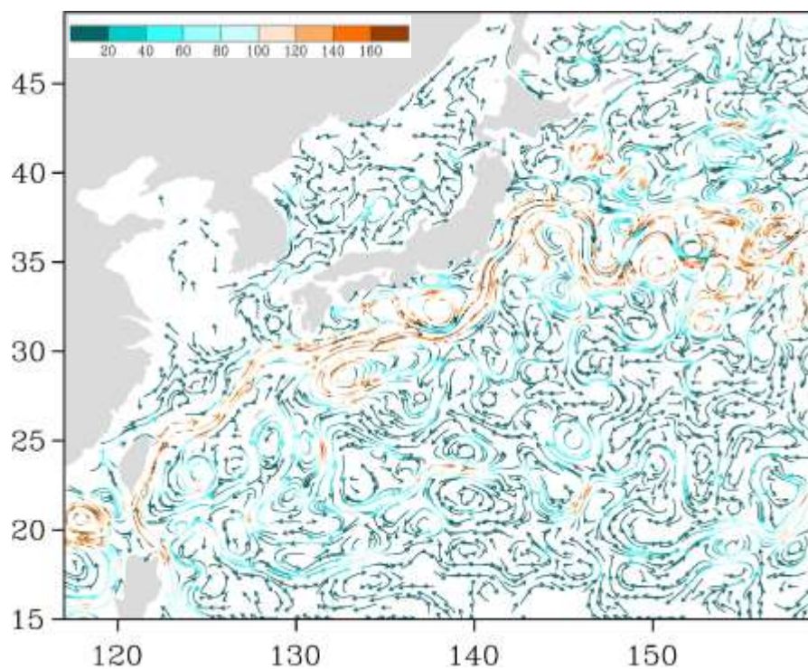
Рис. 3-6 Поверхностные течения западной части Тихого океана, 25 марта 2021 г.
