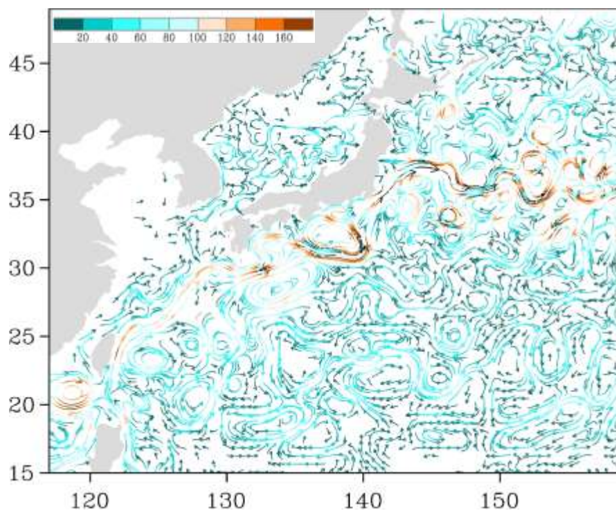
Рис. 3-4 Поверхностные течения западной части Тихого океана, 5 марта 2021 г.
