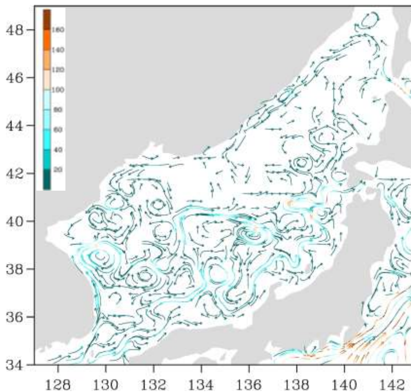
Рис. 3-1 Поверхностные течения Японского моря, 05 марта 2021 г.
