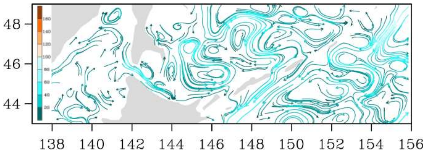
Рис. 3-7 Поверхностные течения, пролив Лаперуза, 5 марта 2021 г.
