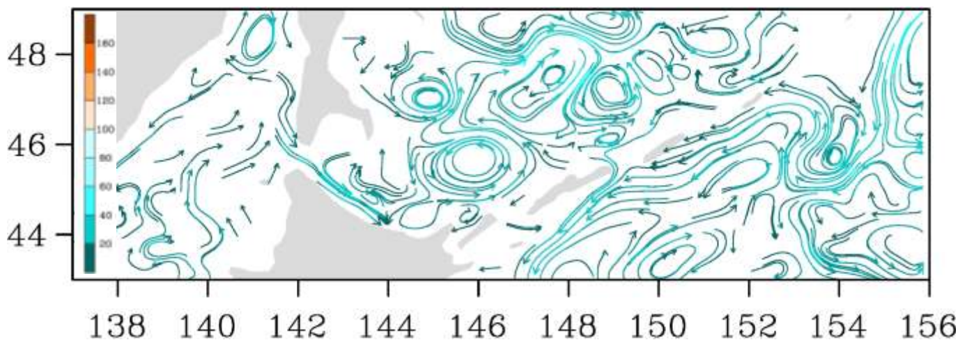
Рис. 3-9 Поверхностные течения, пролив Лаперуза, 25 марта 2021 г.
