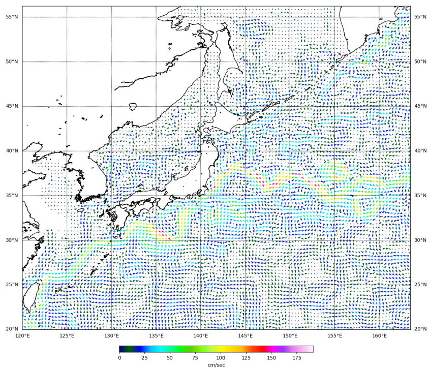
Рис. 3-4 Поверхностные течения западной части Тихого океана, 5 февраля 2023 г.
