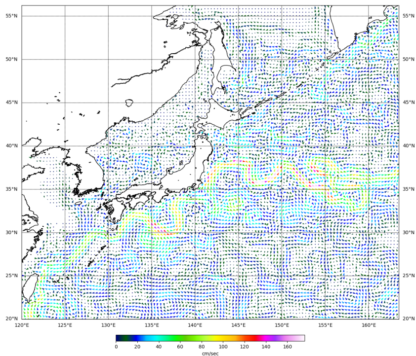
Рис. 3-5 Поверхностные течения западной части Тихого океана, 15 февраля 2023 г.
