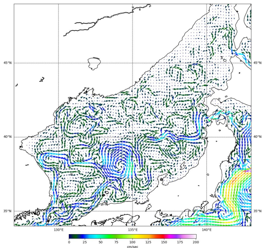
Рис. 3-3 Поверхностные течения Японского моря, 25 февраля 2023 г.
