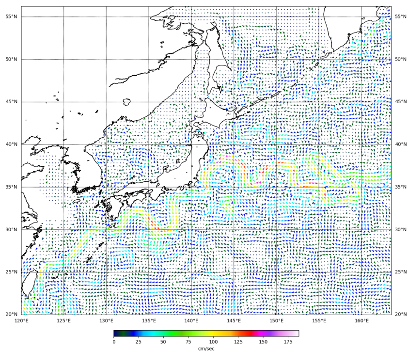
Рис. 3-6 Поверхностные течения западной части Тихого океана, 25 февраля 2023 г.
