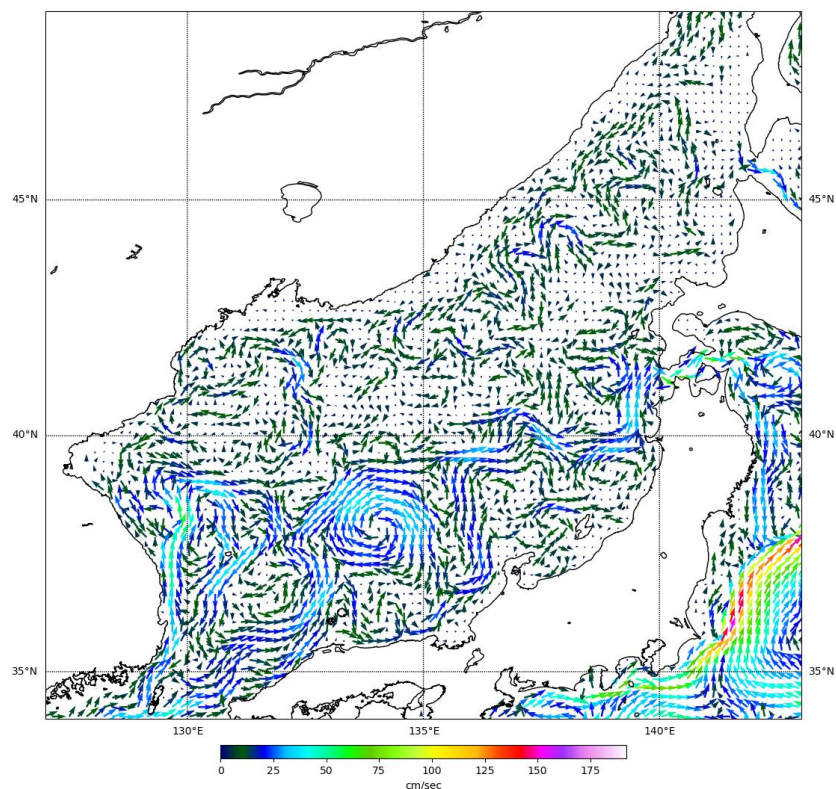
Рис. 3-1 Поверхностные течения Японского моря, 05 февраля 2023 г.
