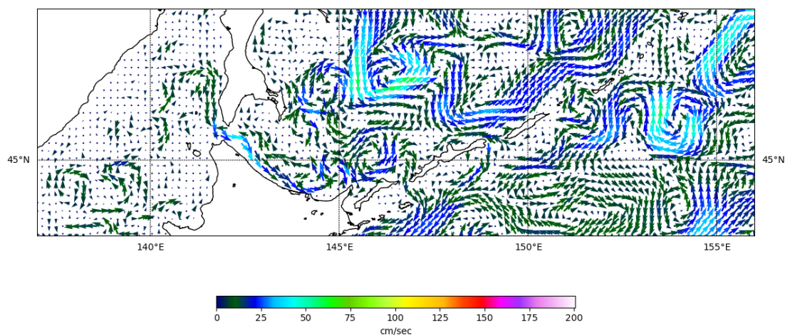
Рис. 3-9 Поверхностные течения, южная часть Охотского моря, 25 февраля 2023 г.
