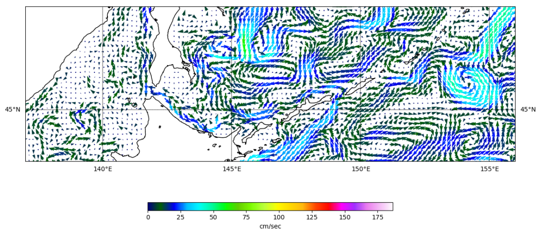
Рис. 3-8 Поверхностные течения, южная часть Охотского моря, 15 февраля 2023 г.
