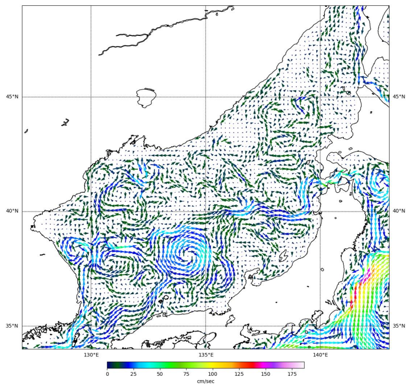
Рис. 3-2 Поверхностные течения Японского моря, 15 февраля 2023 г.
