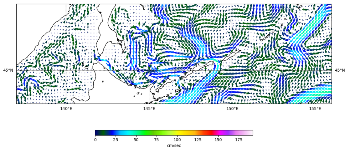
Рис. 3-7 Поверхностные течения, южная часть Охотского моря, 5 февраля 2023 г.
