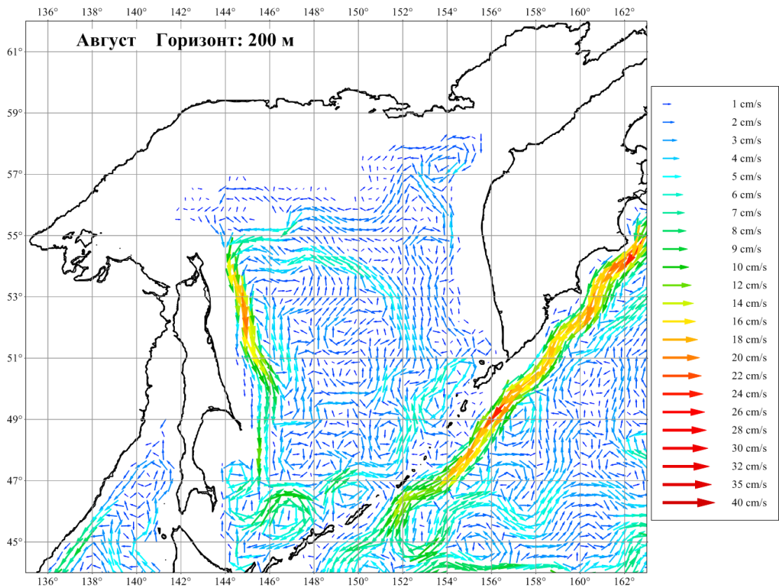
Рисунок 3.48. Течения Охотского моря в августе на горизонте 200 м
