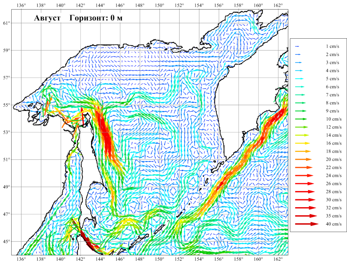
Рисунок 3.44. Течения Охотского моря в августе на горизонте 0 м
