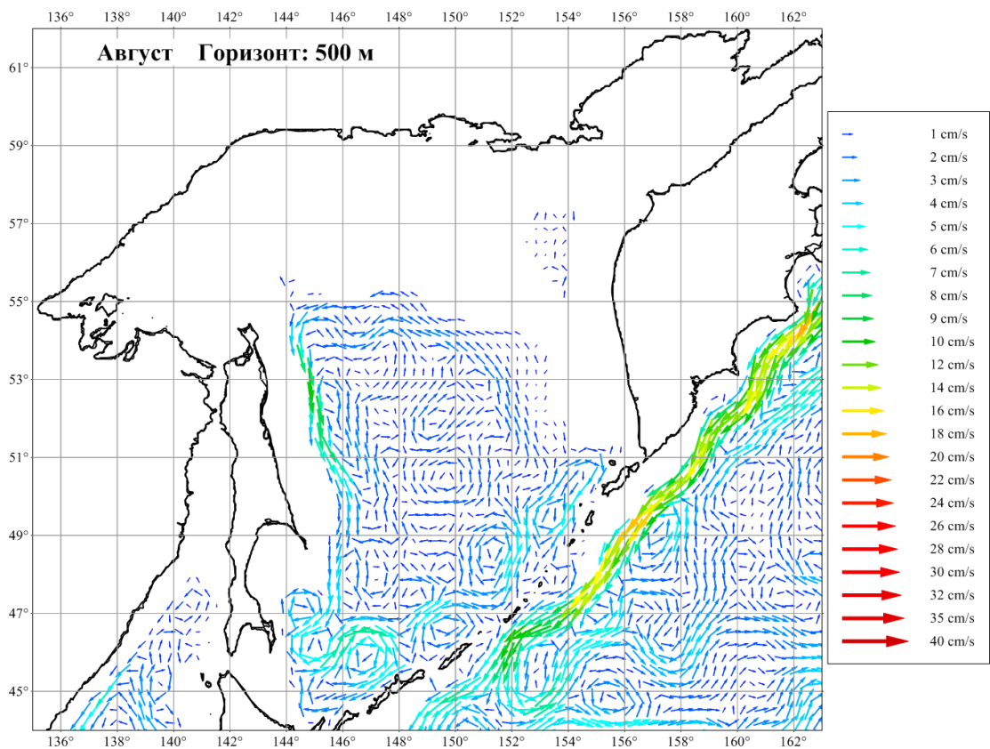
Рисунок 3.49. Течения Охотского моря в августе на горизонте 500 м
