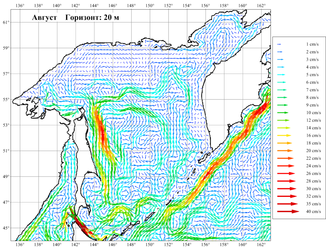
Рисунок 3.45. Течения Охотского моря в августе на горизонте 20 м
