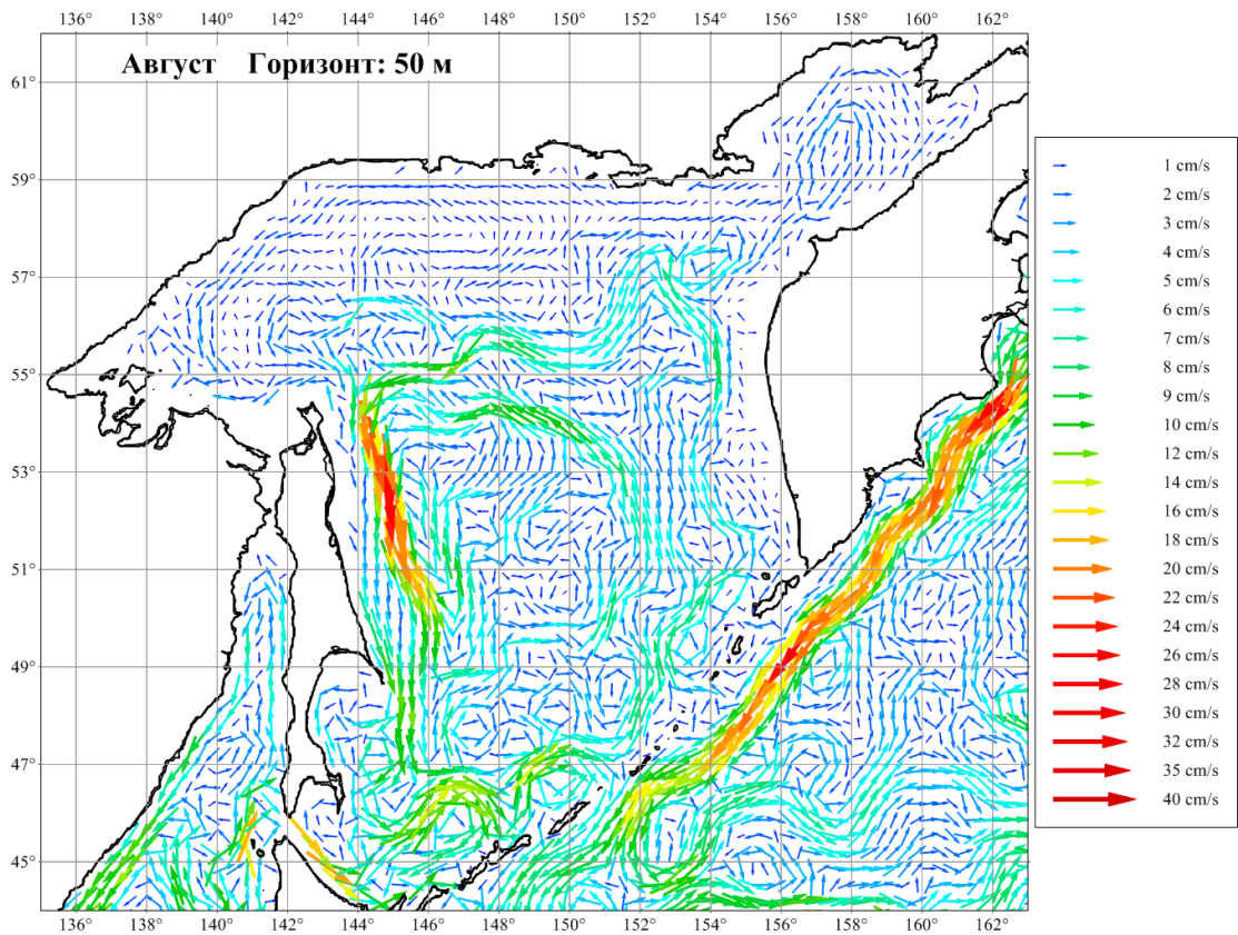
Рисунок 3.46. Течения Охотского моря в августе на горизонте 50 м
