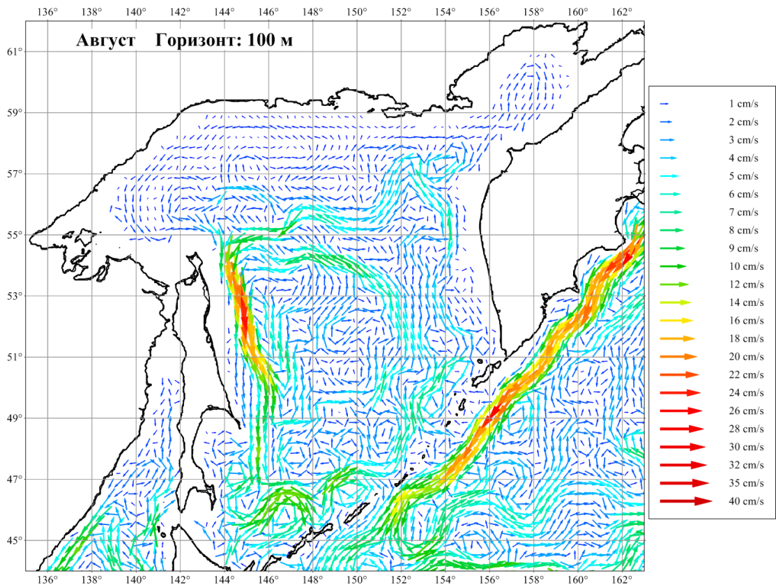
Рисунок 3.47. Течения Охотского моря в августе на горизонте 100 м
