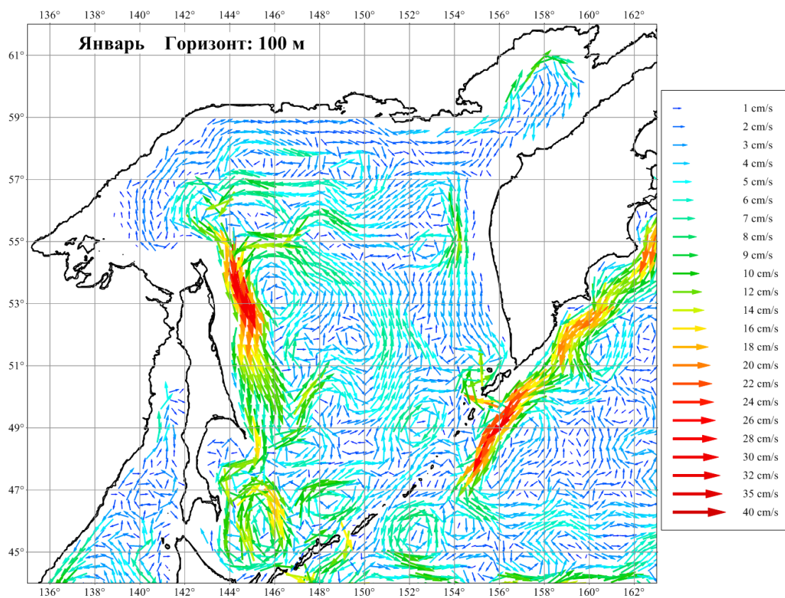
Рисунок 3.5. Течения Охотского моря в январе на горизонте 100 м
