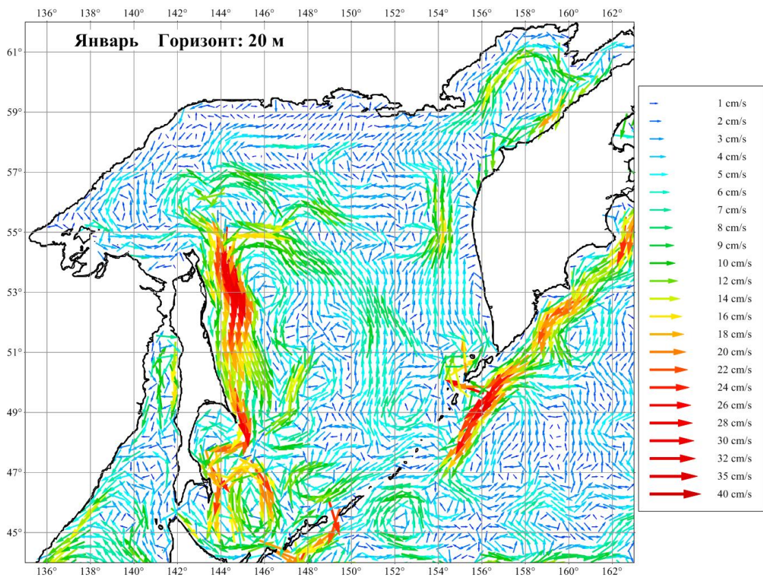
Рисунок 3.3. Течения Охотского моря в январе на горизонте 20 м
