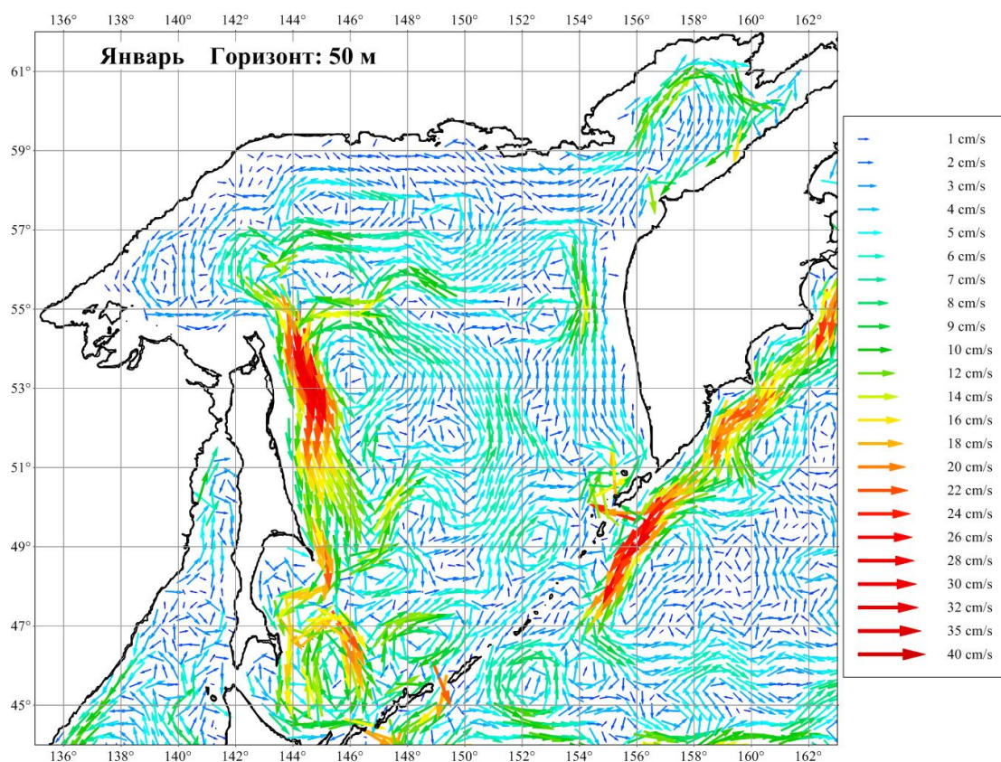
Рисунок 3.4. Течения Охотского моря в январе на горизонте 50 м
