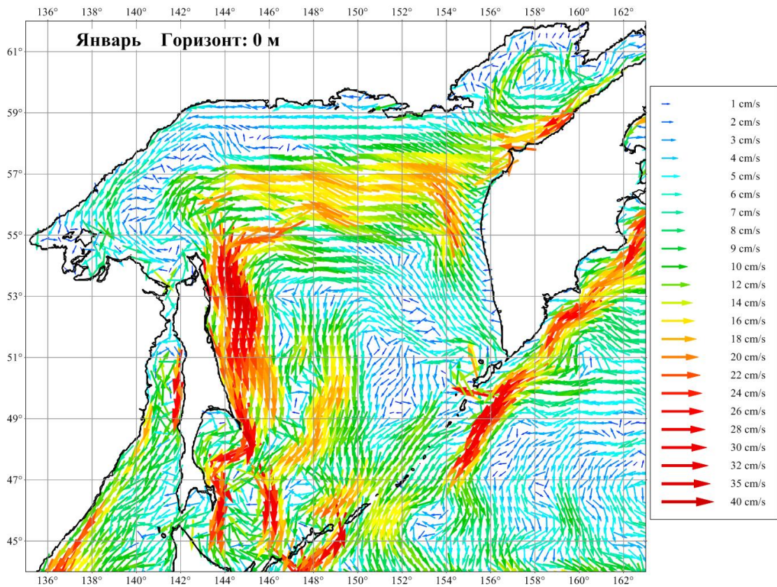
Рисунок 3.2. Течения Охотского моря в январе на горизонте 0 м
