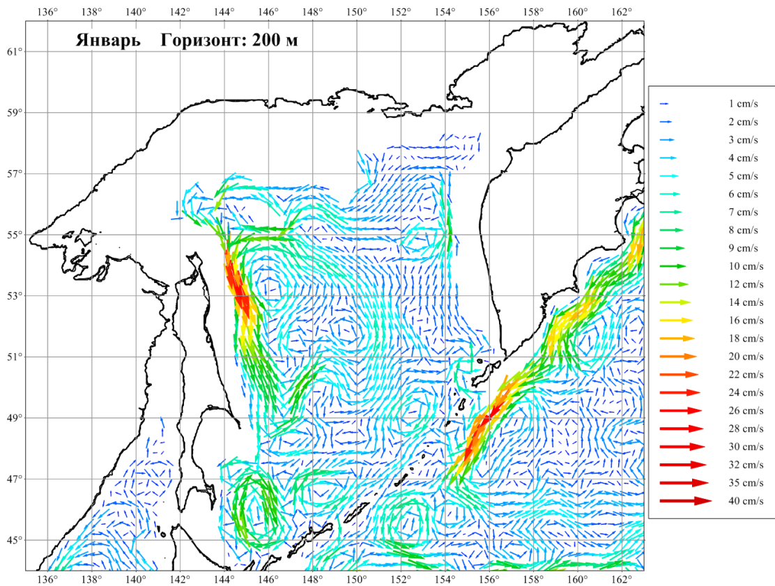
Рисунок 3.6. Течения Охотского моря в январе на горизонте 200 м
