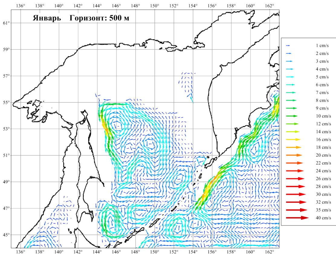
Рисунок 3.7. Течения Охотского моря в январе на горизонте 500 м
