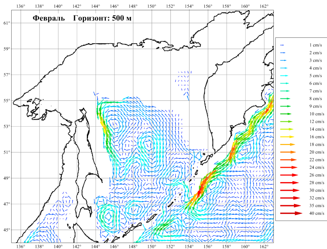
Рисунок 3.13. Течения Охотского моря в феврале на горизонте 500 м
