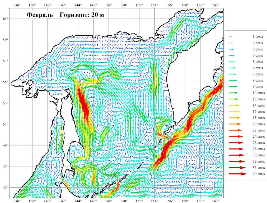
Рисунок 3.9. Течения Охотского моря в феврале на горизонте 20 м
