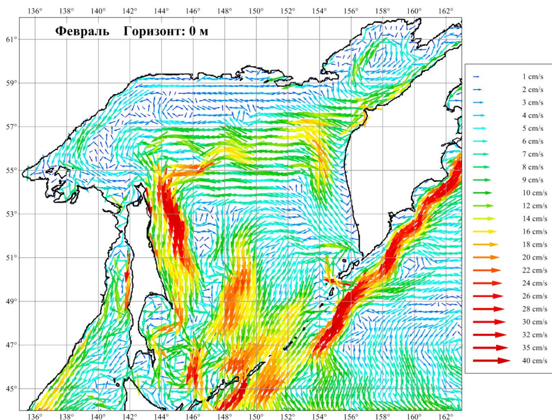
Рисунок 3.8. Течения Охотского моря в феврале на горизонте 0 м
