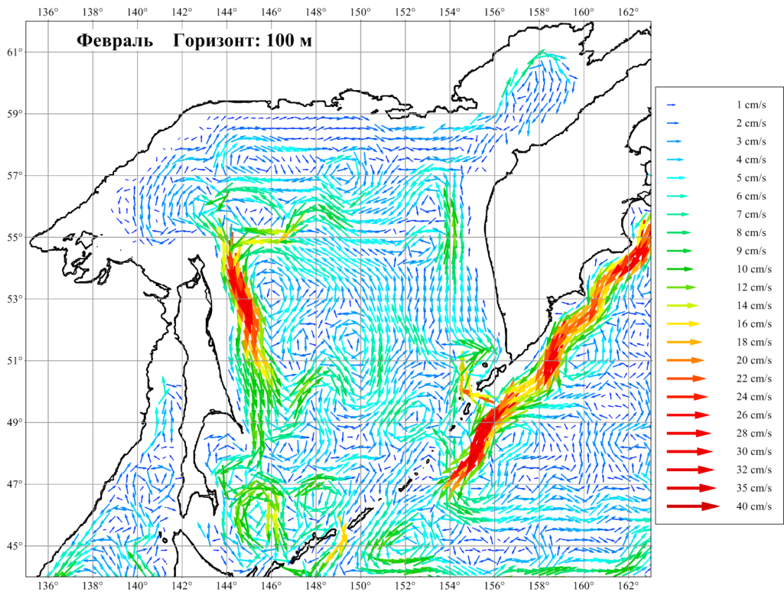
Рисунок 3.11. Течения Охотского моря в феврале на горизонте 100 м
