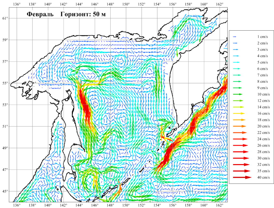
Рисунок 3.10. Течения Охотского моря в феврале на горизонте 50 м
