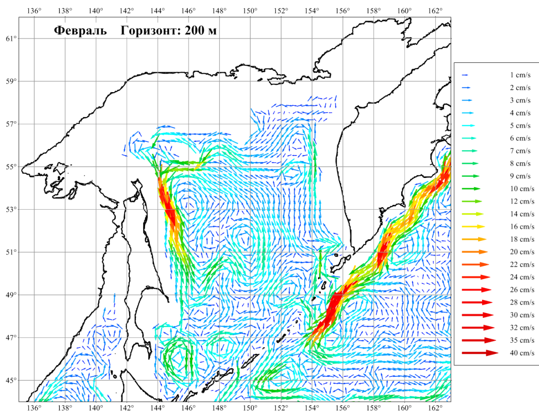
Рисунок 3.12. Течения Охотского моря в феврале на горизонте 200 м
