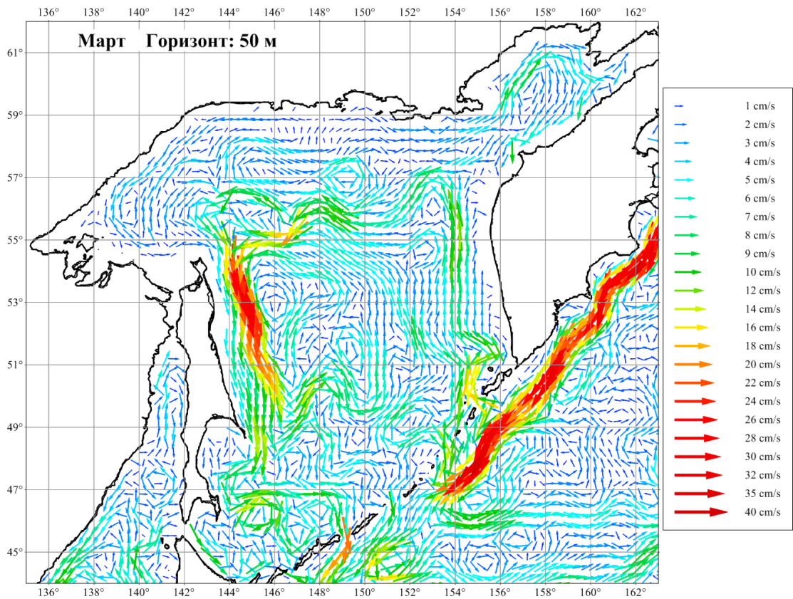
Рисунок 3.16. Течения Охотского моря в марте на горизонте 50 м
