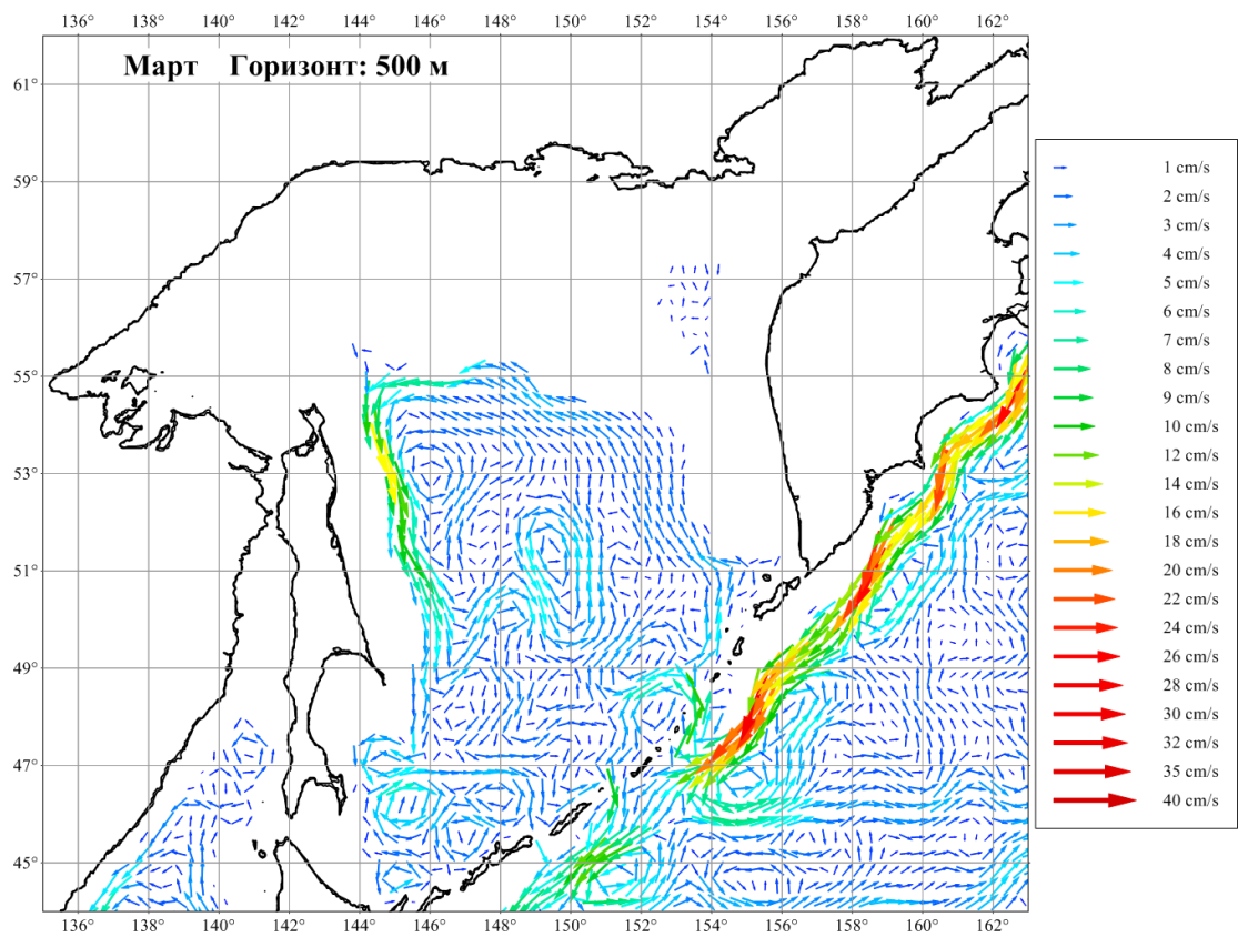
Рисунок 3.19. Течения Охотского моря в марте на горизонте 500 м
