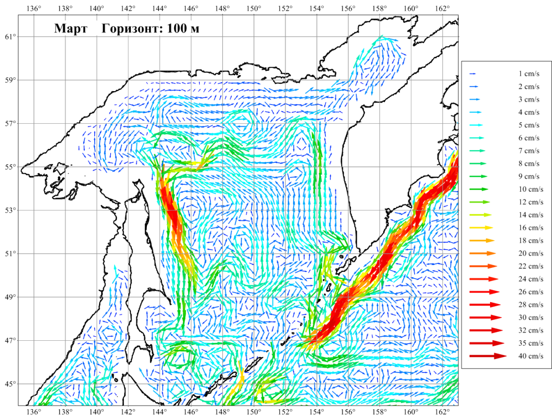
Рисунок 3.17. Течения Охотского моря в марте на горизонте 100 м
