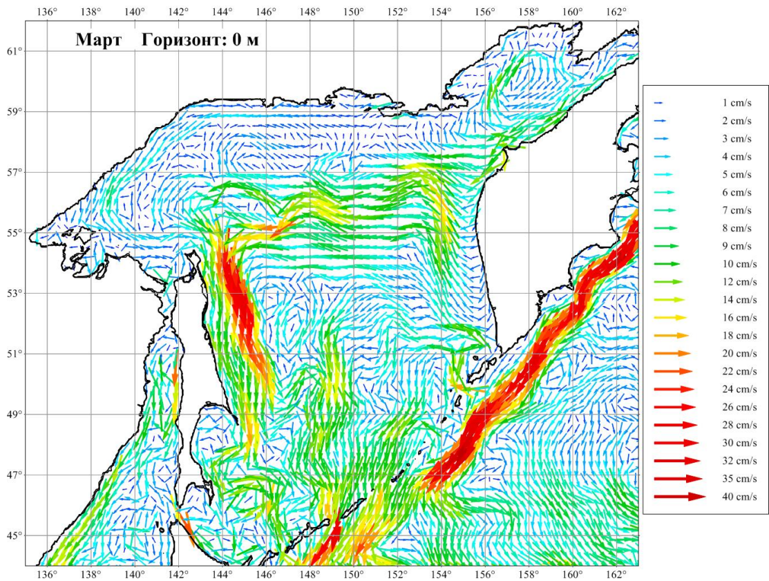
Рисунок 3.14. Течения Охотского моря в марте на горизонте 0 м
