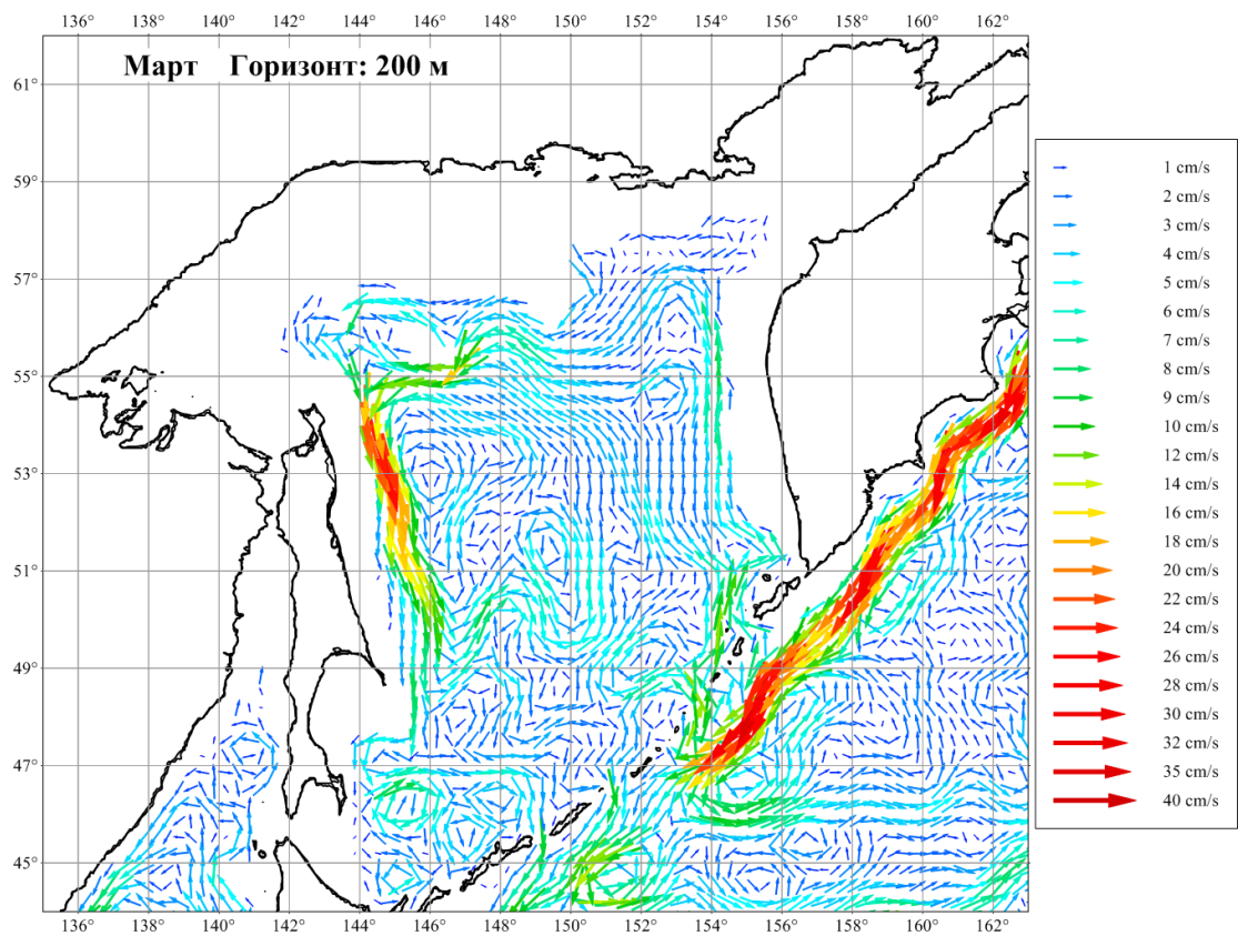
Рисунок 3.18. Течения Охотского моря в марте на горизонте 200 м
