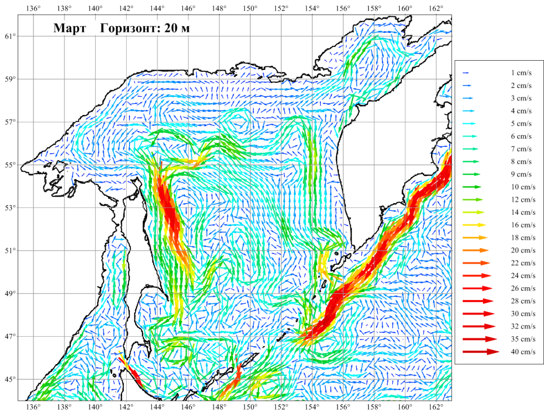
Рисунок 3.15. Течения Охотского моря в марте на горизонте 20 м
